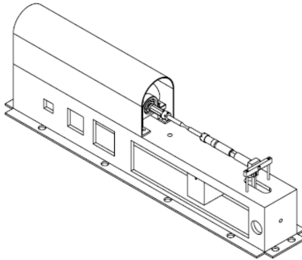
Figura 1. Máquina a fatiga en estudio.
