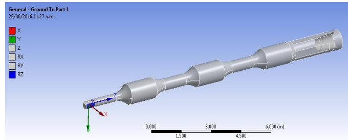
Figura 3. Condiciones frontera para el lado del acoplamiento.
