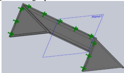
Figura 3. Condiciones de Frontera en la Base
