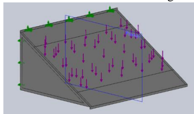
Figura 4. Carga aplicada equivalente a 180 kg
