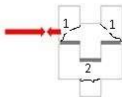
Figura 2. Zonas de posible rompimiento de la pieza.
