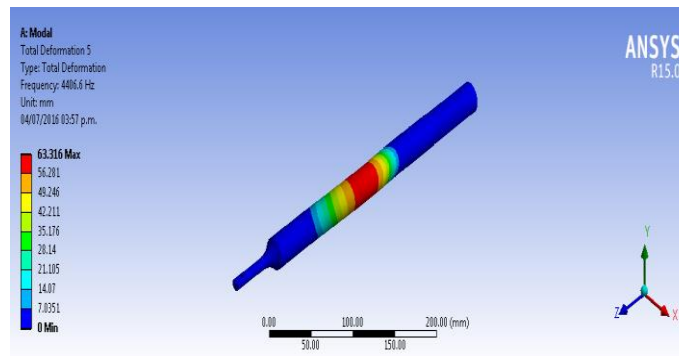
Figura 11. Forma de vibrar cinco en flexión del eje.
