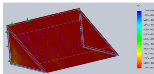
Figura 11. Factor de Seguridad
