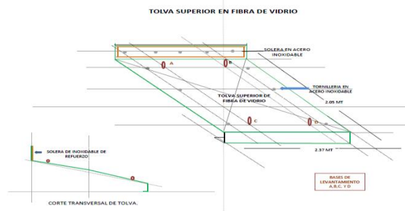
Figura 2. Medidas de una ménsula
