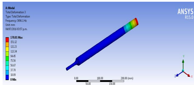
Figura 10. Forma de vibrar uno en flexión coladizo del eje modificado.
