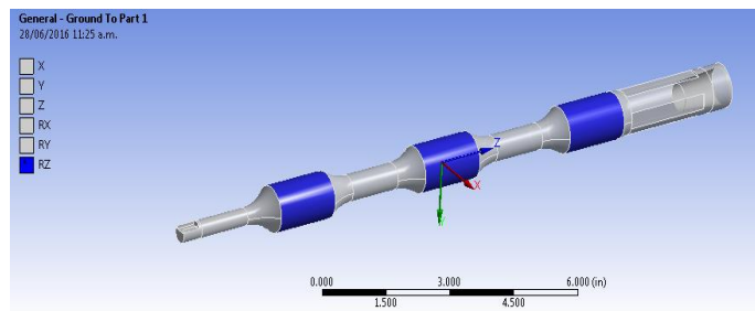
Figura 2. Condiciones frontera para chumaceras.
