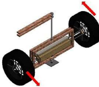
Figura 5. Prensa para fabricar piezas de BTC
