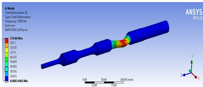
Figura 6. Forma de vibrar entre dos chumaceras.
