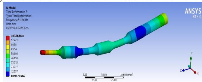
Figura 7. Forma de vibrar en condición libre-libre del eje.
