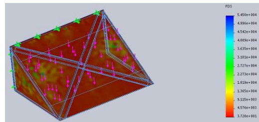
Figura 14. Factor de Seguridad
