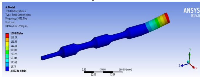
Figura 4. Forma de vibrar en voladizo.
