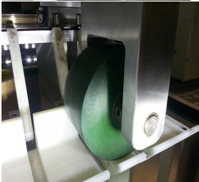
Figura 6. Rodillo nuevo con un diseño mejorado para aplicación de Maylar y evitar la formación de burbujas.
