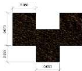
Figura 3. Dimensiones del BTC propuesto.
