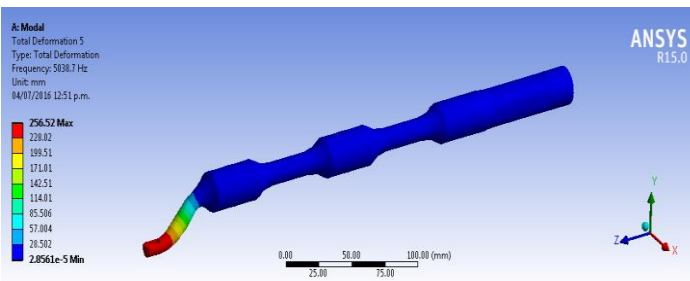
Figura 5. Forma de vibrar del lado del acoplamiento.
