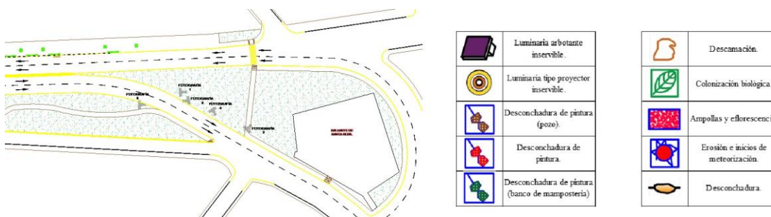
Figura 3. Plano y extracto de la simbología de deterioros, figura izquierda de la vialidad, figura derecha del inmueble, Fuente: Propia (2018).
