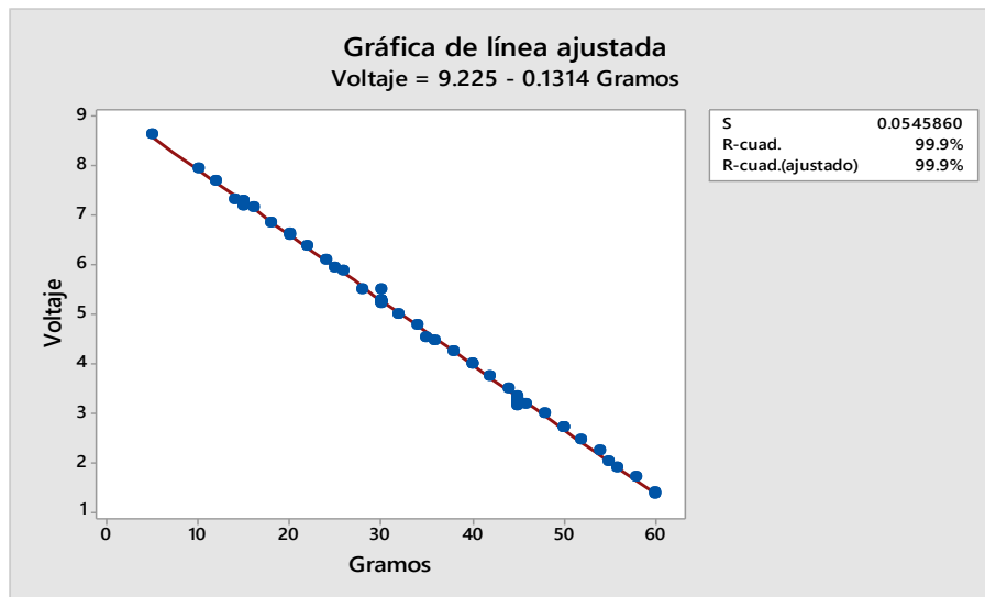
Figura 1. Grafica de regresión lineal, indicando la relación del voltaje con el peso en gramos.
