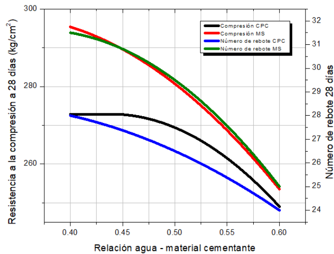
Figura 7. Correlación entre f'c y número de rebote, en función de la relación a/mc
