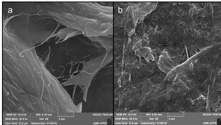
Figura 5. Microscopía electrónica de barrido: a) MFLC y b) MFC.
