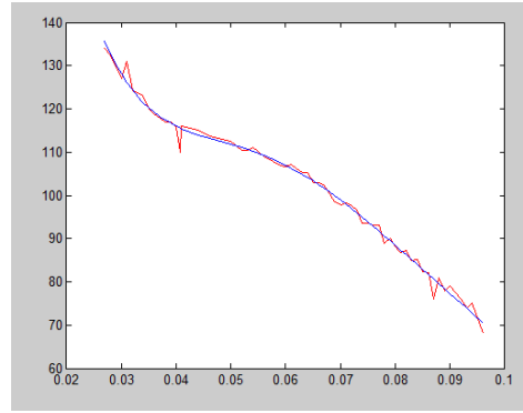
Figura 4. Gráfica de la relación de la glucosa con respecto del voltaje junto con la evaluación de todos los voltajes en el polinomio.
