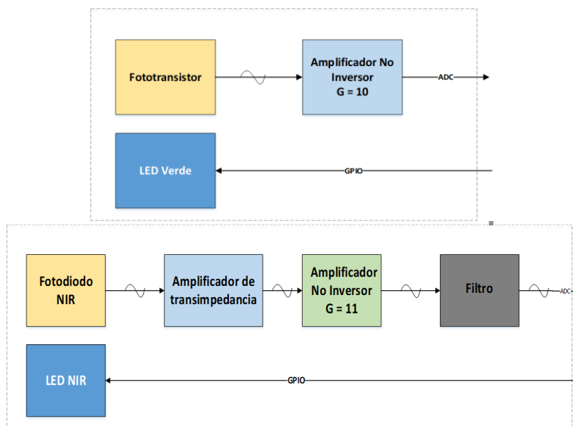
Figura 1. Esquema general del sistema no invasivo de medición de glucosa.
