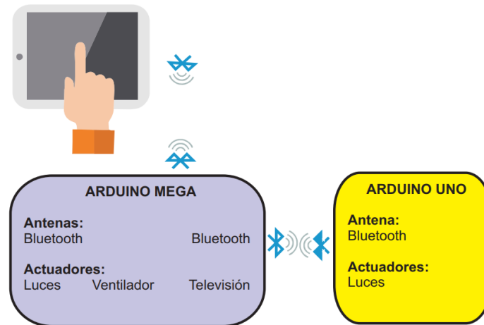
Figura 1. Esquema del prototipo.
