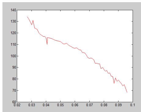
Figura 3. Gráfica de la relación de la glucosa con respecto del voltaje.
