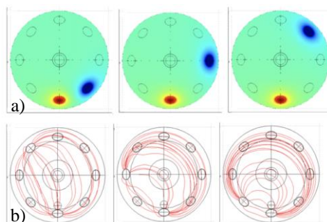
Figura 3. Representación del electrodo de inyección en este caso el 1 y de referencia, así como las líneas del campo eléctrico.
