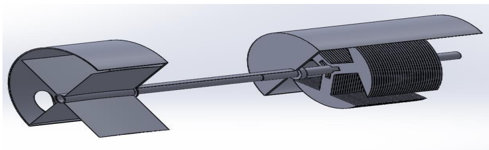
Figura No.2 Componentes de la caldera piro-tubular.
