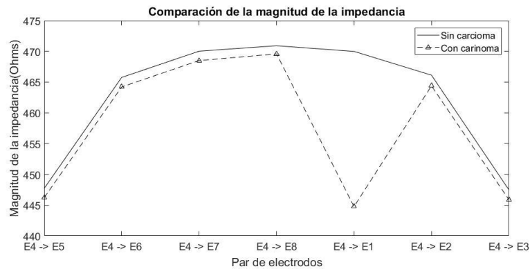
Figura 6. Comparación de la impedancia sin carcinoma y con carcinoma.
