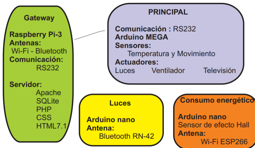
Figura 6. Esquema de la versión final del proyecto.
