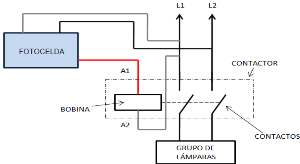
Figura 3. Ejemplo de conexión de fotocelda para control de contactor.
