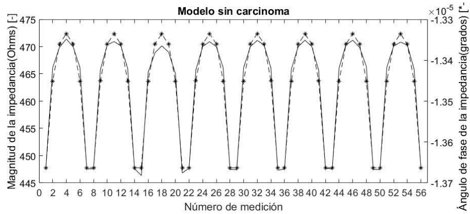
Figura 4. La EIS obtenidas de la simulación de una mama sin carcinoma.
