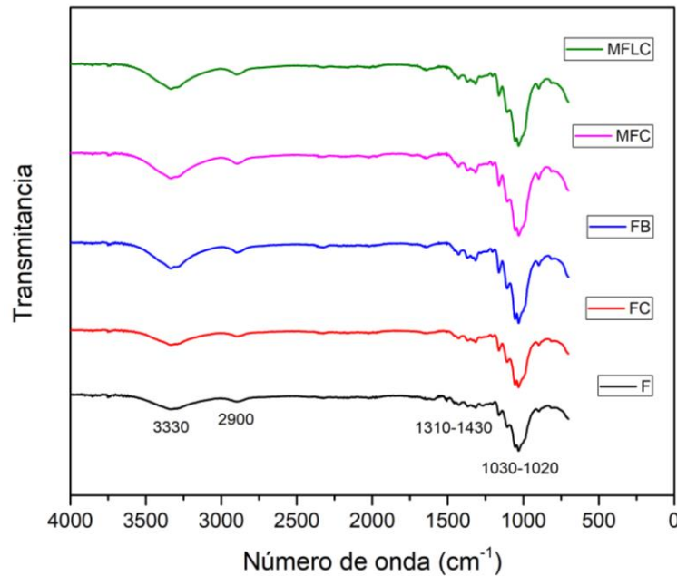
Figura 6. Espectroscopía Infrarroja FTIR-ATR de F, FC, FB, MFC y MFLC.
