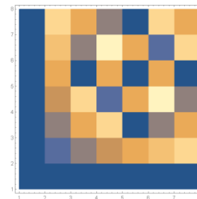
Figura 2. Multiplicación en \mathbb{Z}_8
