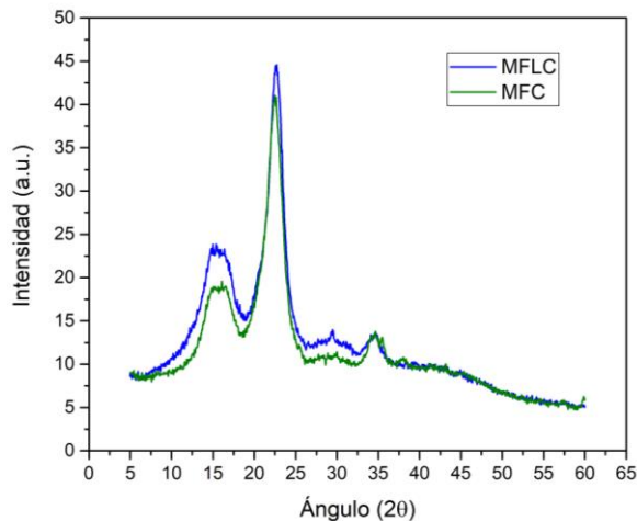
Figura 7. Difracción de rayos X de MFLC y MFC.
