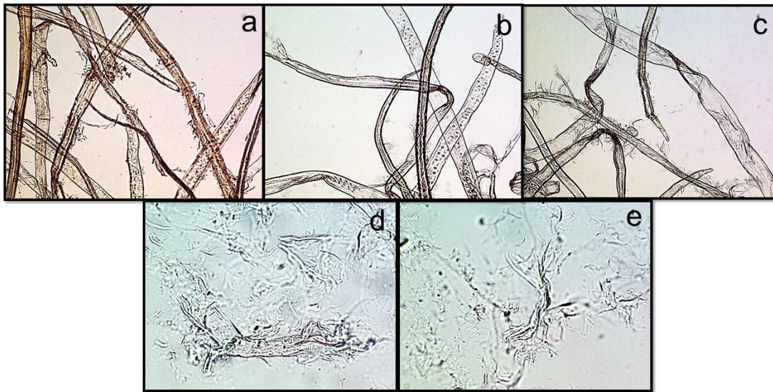
Figura 3. Microscopía óptica de pulpas de cartón OCC: a) F-OCC 10X, b) FC-OCC 10X, c) FB-OCC 40X, d) MFLC-OCC 40X, e) MFC-OCC 40X.
