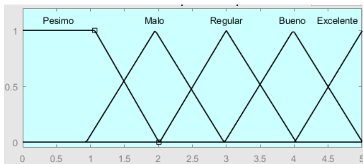
Figura 1. Conjuntos difusos.
