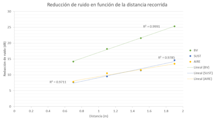
Figura 3: reducción de sonido comparación entre la barrera verde, el sustrato de tezontle y el aire
