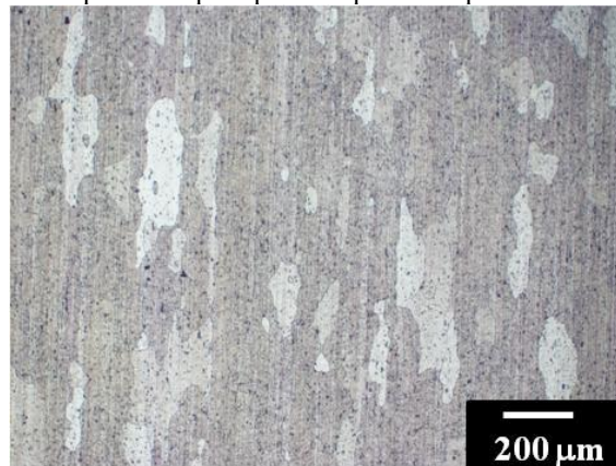
Figura 3: Microestructura del metal base en condición de llegada.
