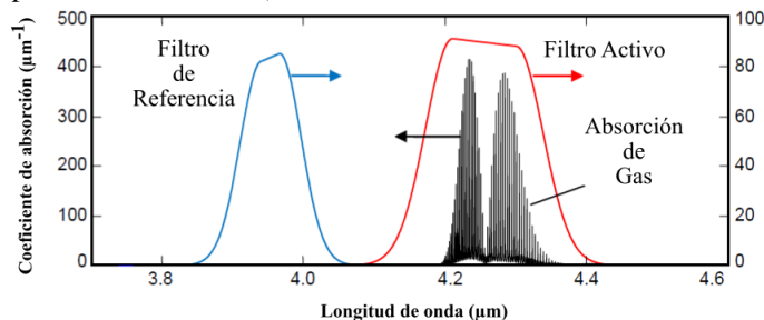
Figura 1. Principio de medición NDIR para la medición de CO 2 .
