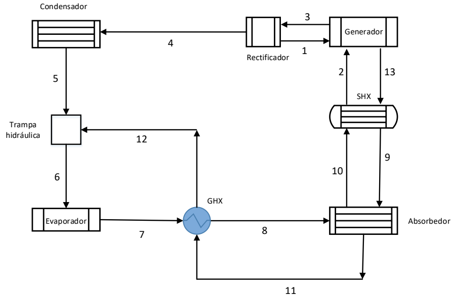
Figura 1. Diagrama esquemático de un sistema de refrigeración difusión-absorción.
