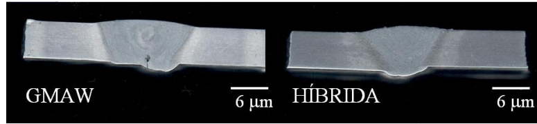
Figura 4: Perfil transversal de la macroestructura de las uniones soldadas.
