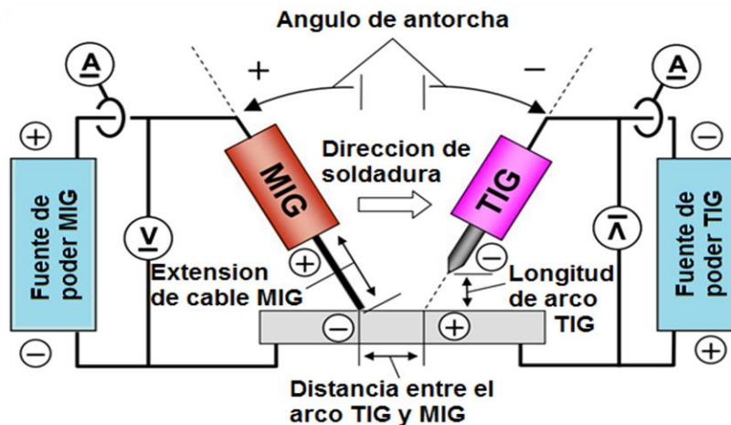
Figura 1. Esquema del proceso de soldadura híbrido GTAW-GMAW. Modificado de Kanemaru, Shuhei, et al (2014)
