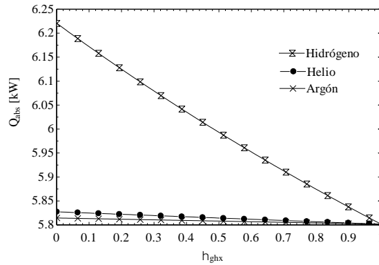
Figura 4. Efecto de la efectividad del GHX sobre el calor del absorbedor
