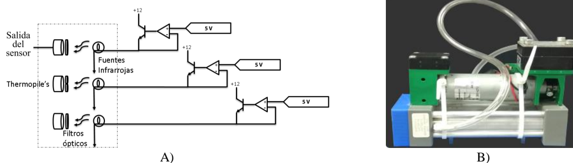
Figura 5. Cámara de gases para medir CO, CO 2 y HC, su estructura general mostrado en A) y el empleo en el sistema.
