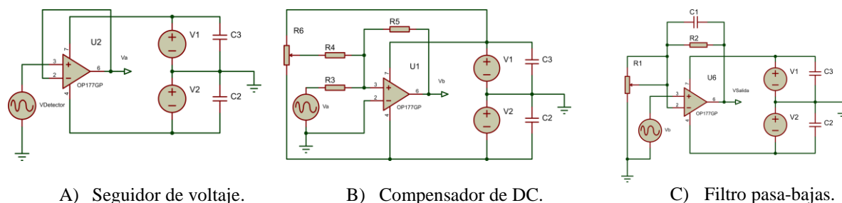
Figura 6. Circuitos electrónicos que componen la instrumentación del sensor 2M Quad para medir los gases.
