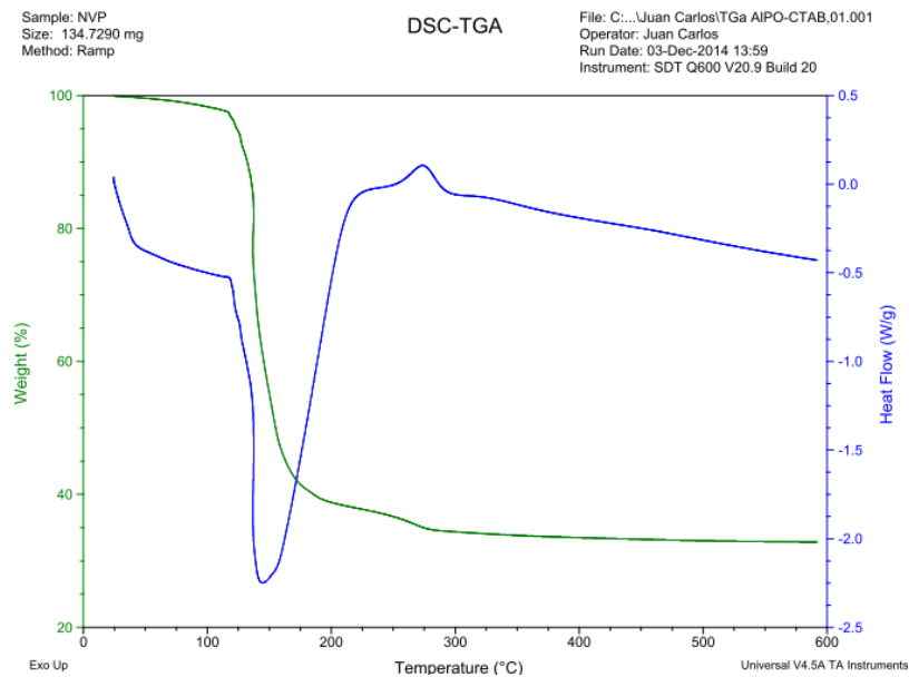
Figura 2. Análisis de TGA para las soluciones de CTAB/AIPO
