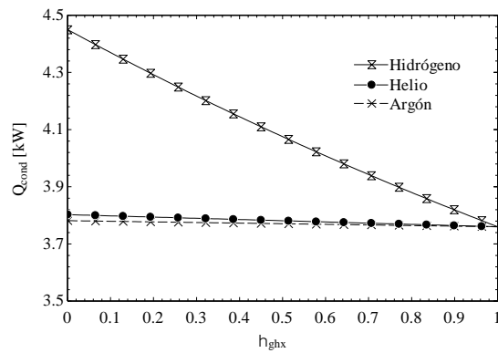
Figura 5. Efecto de la efectividad del GHX sobre el calor del condensador
