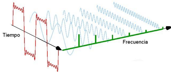
Figura 1. Espectro de amplitud de una función f(t) .
