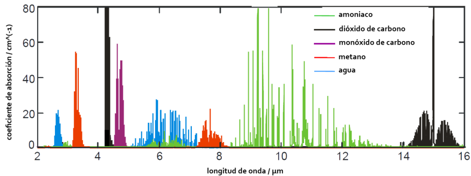
Figura 3. Espectro de absorción para cinco gases en la región media infrarroja del espectro.
