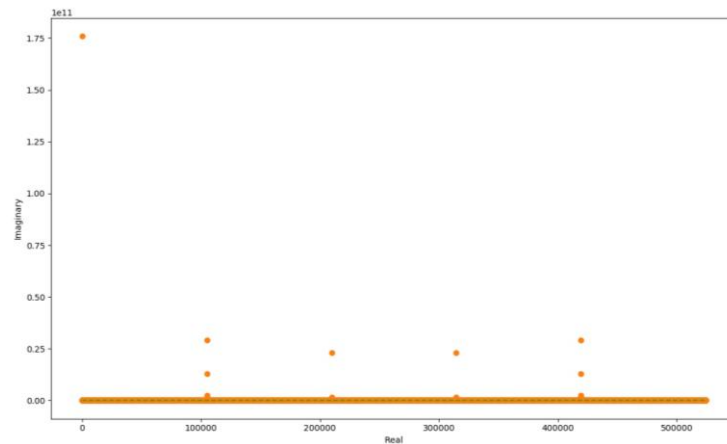
Figura 3. Espectro de magnitud para el juego (2, 7, 8)-Nim.
