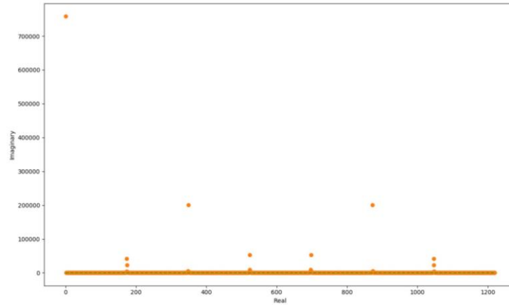
Figura 2. Espectro de magnitud para el juego (2, 5)-Nim.
