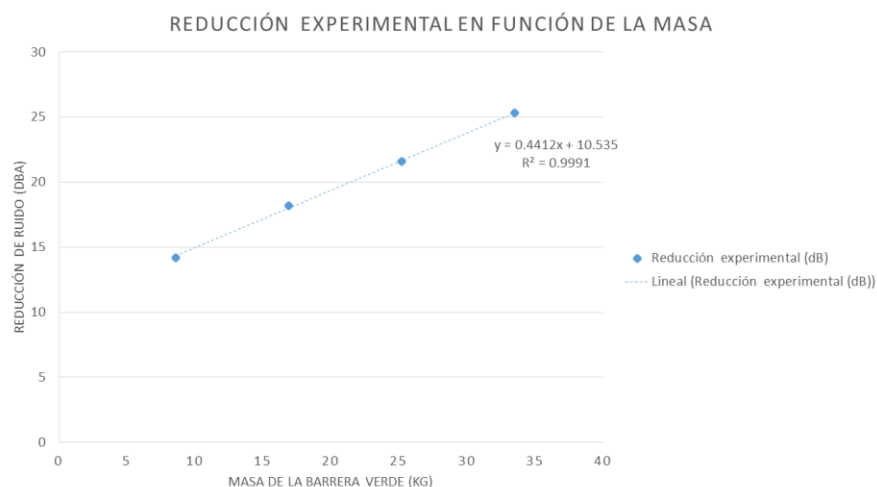
Figura 4: Reducción de ruido en función de la masa de la barrera verde. La masa de la barrera verde incluye la biomasa de las plantas y el aire atrapado entre las mismas.
