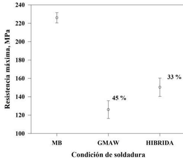
Figura 8: Gráfica de la pérdida de la resistencia máxima del proceso de soldadura GMAW y el proceso de soldadura híbrida con respecto al metal base. GMAW pérdida del 45% e HÍBRIDA pérdida del 33%.
