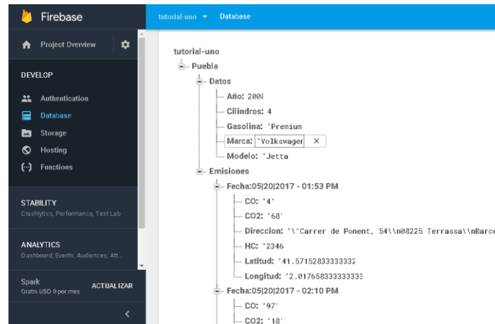
Figura 2. Interfaz Web para Firebase, muestra los datos del usuario y emisiones de nuestro sistema en formato JSON.
