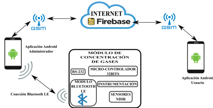
Figura 1. Arquitectura del sistema para la medición de gases de CO, CO 2 y HC.
