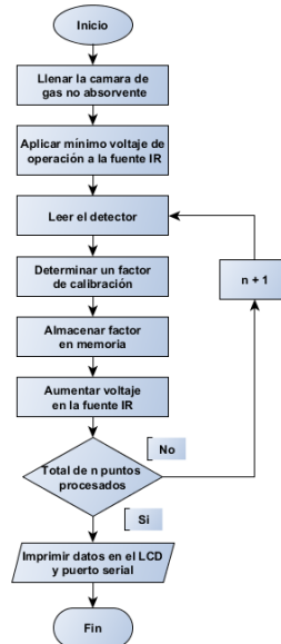
Figura 7. Diagrama de flujo de la digitalización y calibración.
