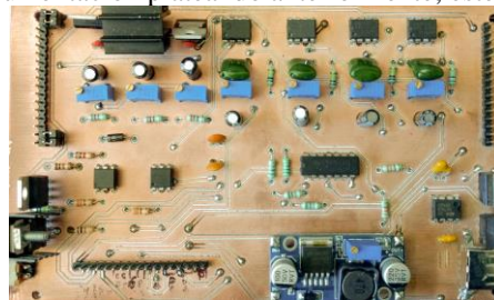
Figura 8. Circuito impreso de las etapas de compensación, amplificación y filtrado.
