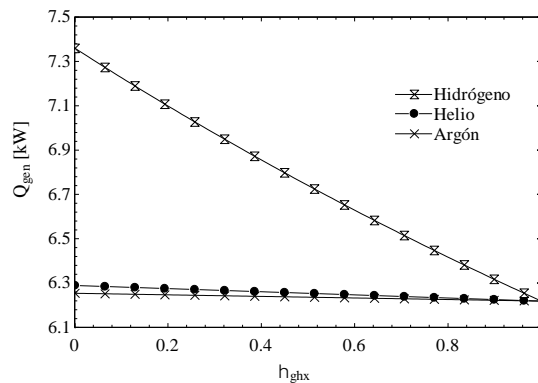
Figura 3. Efecto de la efectividad del GHX sobre el calor del generador
