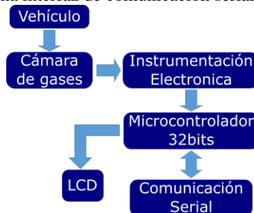
Figura 4. Diagrama del sistema para medir CO, CO 2 y HC.
