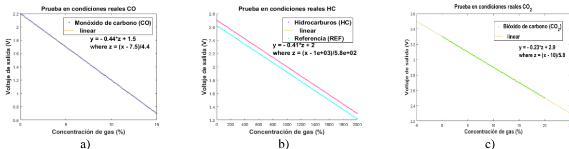
Figura 9. Gráficas de concentración de los gases CO, CO 2 y HC vs voltaje correspondientemente a las figuras a), b) y c), a una temperatura de 35° C.
