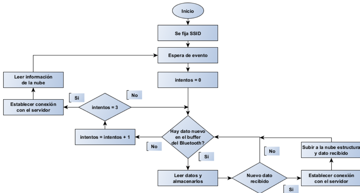
Figura 3. Diagrama de flujo de la aplicación.
