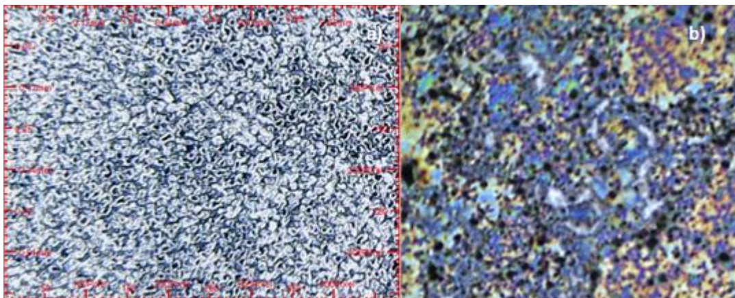
Figura 3. Imagen óptica (a) e imagen por elipsometría (b) del recubrimiento de AIPO sin CTAB.
