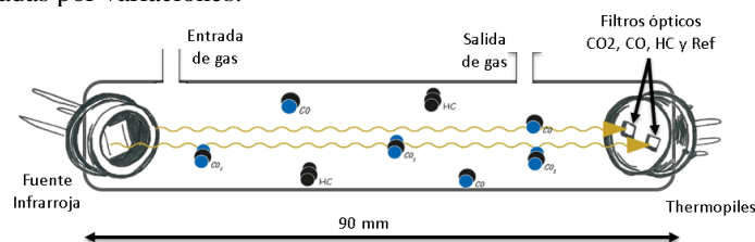
Figura 2. Diagrama esquemático de un típico sensor de gas no dispersivo.
