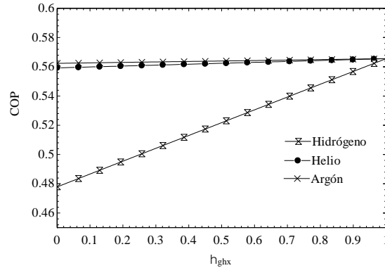
Figura 2. Efecto de la efectividad del GHX sobre el COP
