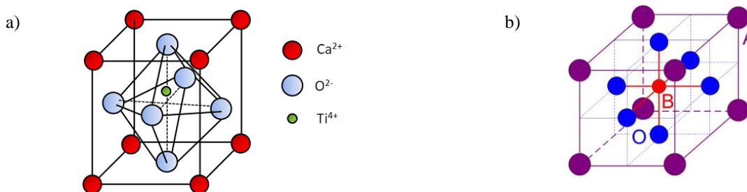
Figura 1. a) Estructura del \text{CaTiO}_3 8 , b) Estructura del tipo perovskita.
