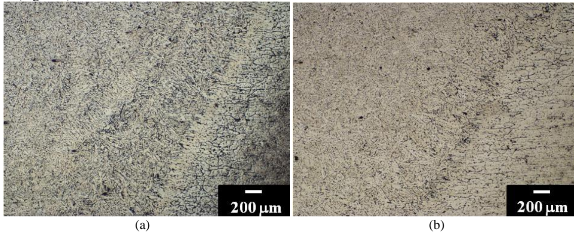
Figura 5: Microestructuras de la ZF y la LF de las muestras soldadas por el proceso de soldadura GMAW y el proceso híbrido de soldadura GTAW-GMAW. (a) Micrografía de la muestra soldada por GMAW a 5x, (b) micrografía de la muestra soldada por el proceso híbrido a 5X
