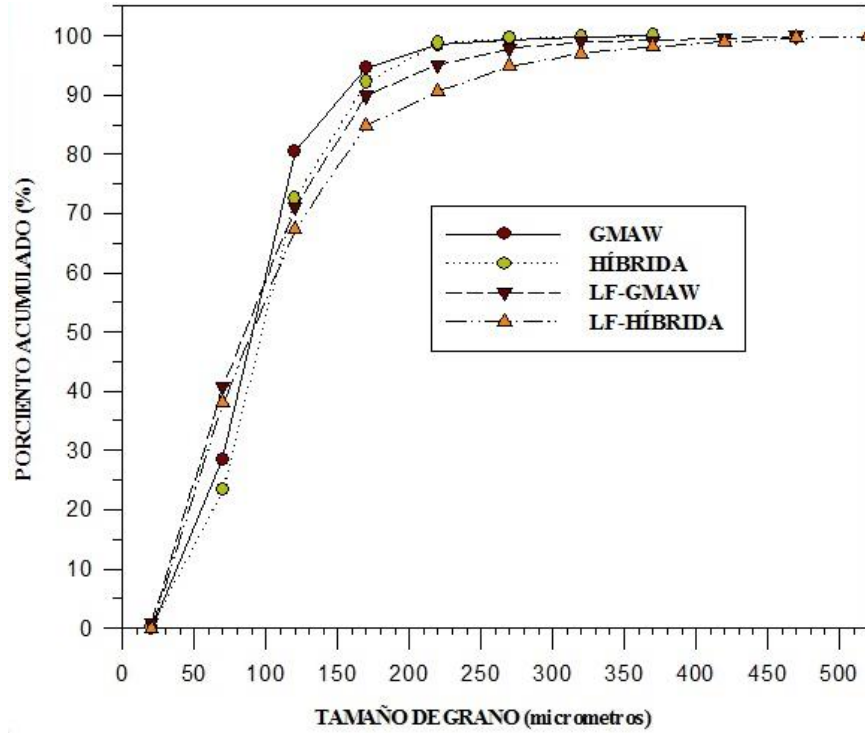
Figura 6: Porcentaje acumulado de las mediciones de tamaño de grano.
