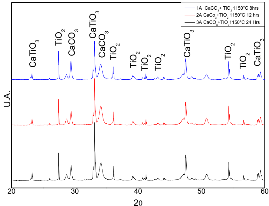
Figura 2. Patrones de difracción de la reacción del óxido de titanio con carbonato de calcio grado reactivo a la temperatura de 1150°C a 8, 12 y 24 horas de permanencia
