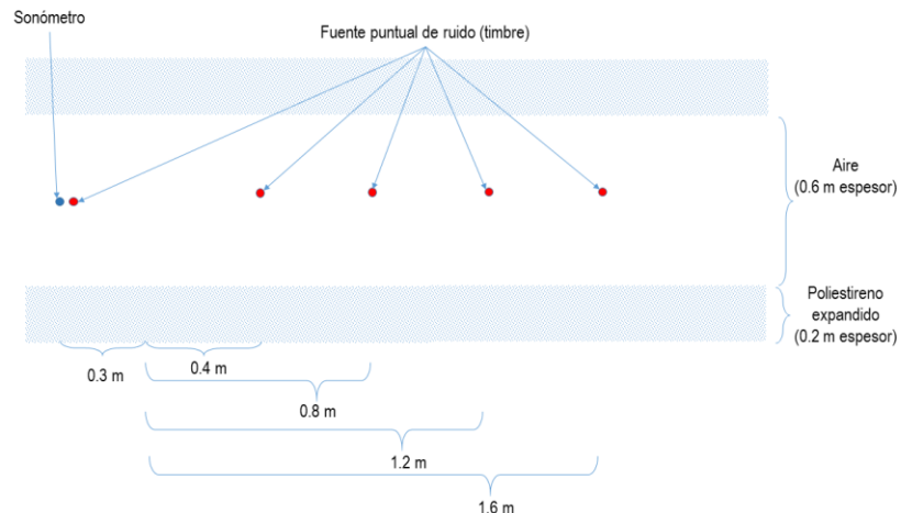
Figura 2. Prototipo para medición de amortiguamiento de
