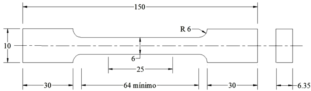
Figura 2: Preparación de las probetas para realizar las prueba de tensión.
