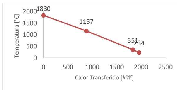
Figura 4.- Relación entre la temperatura y el calor transferido en los pasos
