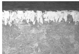
Imagen 1.3. Capa borurada en 6 hrs., y 950 °C a 200X. 10µm.
