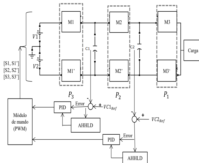
Figura 3. Esquema de la implementación del algoritmo en el convertidor de energía multicelular de tres células.
