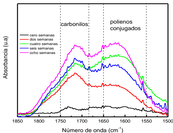
Figura 3.- Espectros de FTIR de tubería de CPVC expuesta a envejecimiento acelerado en la zona de carbonilos
