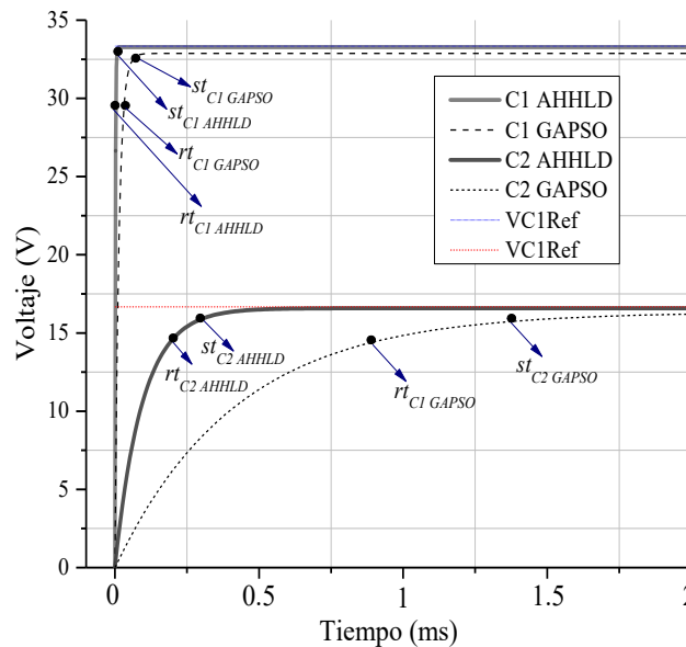
Figura 4. Curvas de respuesta en voltaje de los capacitores flotados C1 y C2.
