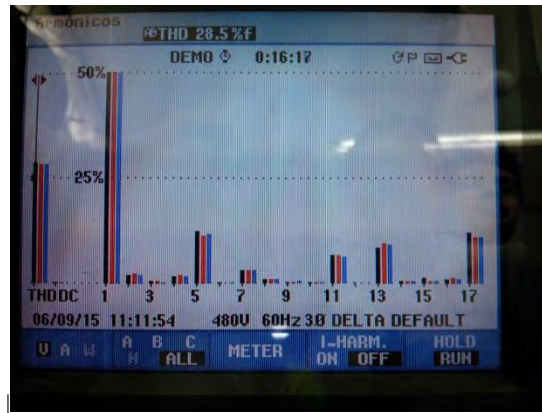
Figura 5. Lectura con el Analizador Fluke 434 en una señal trifásica
