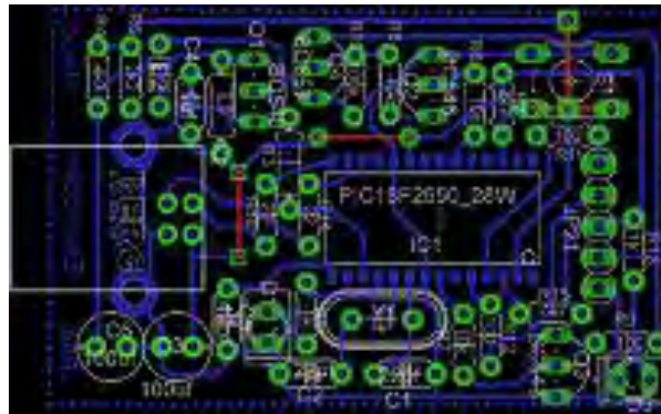
Figura 4. Diseño PCB del Programador Propuesto.
