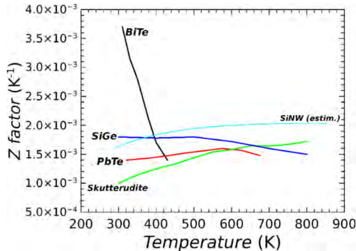
Figura 1. Figura de Mérito Dependiente de la Temperatura
