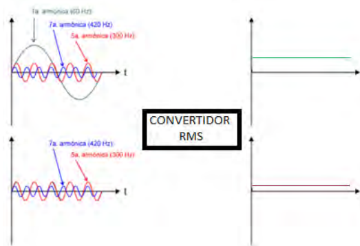
Figura 7. Convertidor RMS
