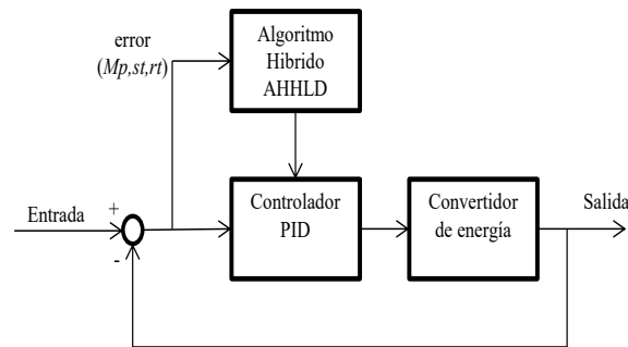
Figura1. Diagrama a bloques de la implementación del algoritmo en el sistema de control.
