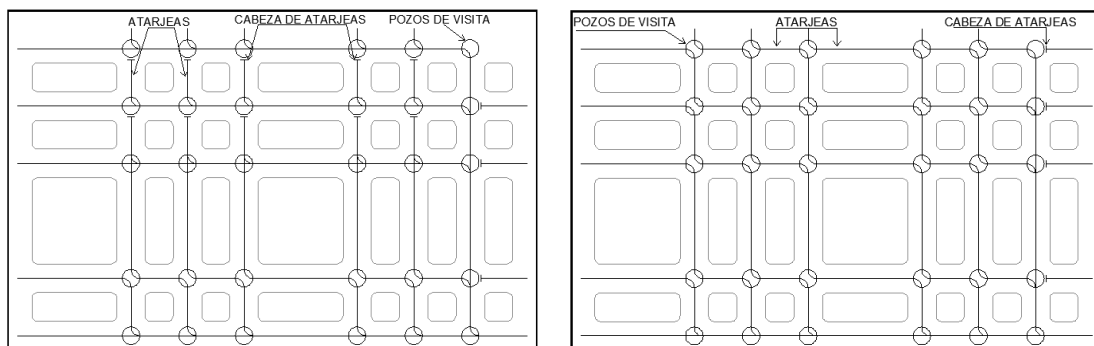
Figura 2. Trazo de la red de atarjeas en Doble Peine (izquierda) y Bayoneta (derecha).
