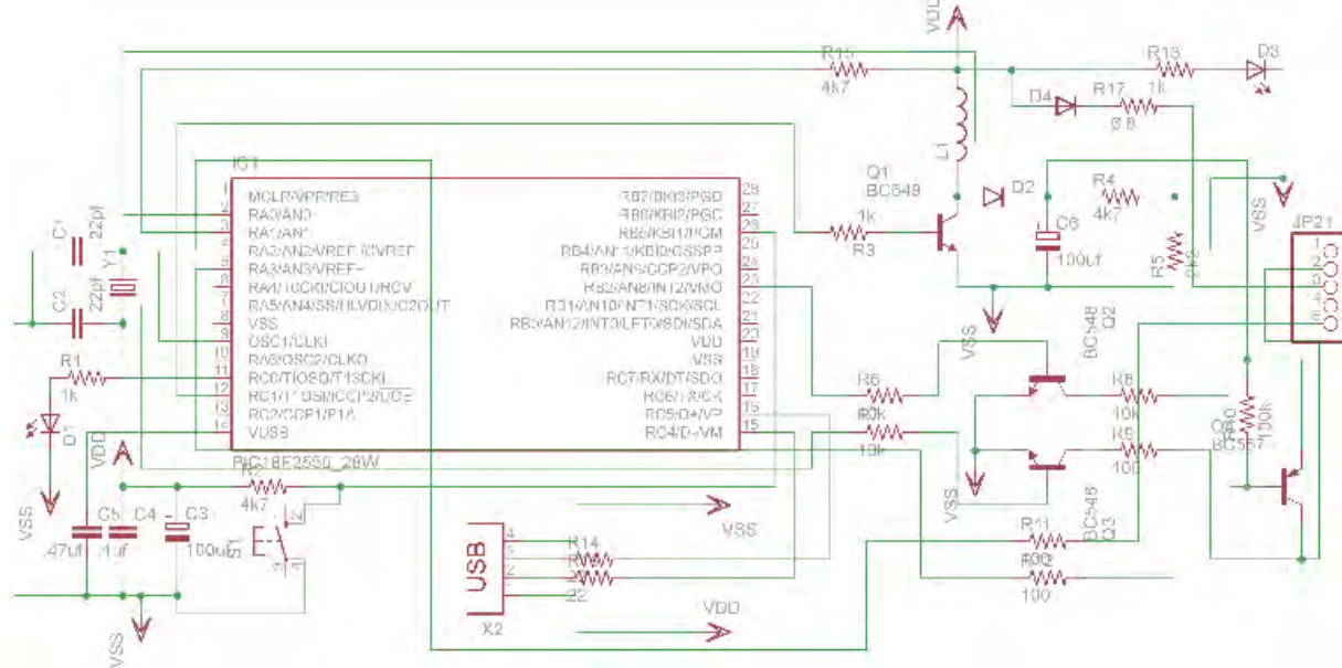
Figura 2. Diagrama Eléctrico del Programador Propuesto
