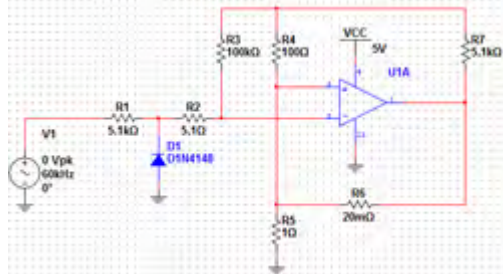
Figura 5 Diagrama de detector de Cruce por cero
