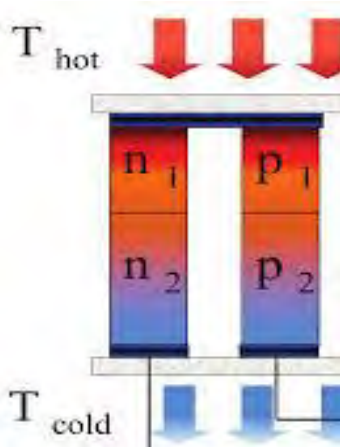
Figura 2. Esquema TEG Segmentado
