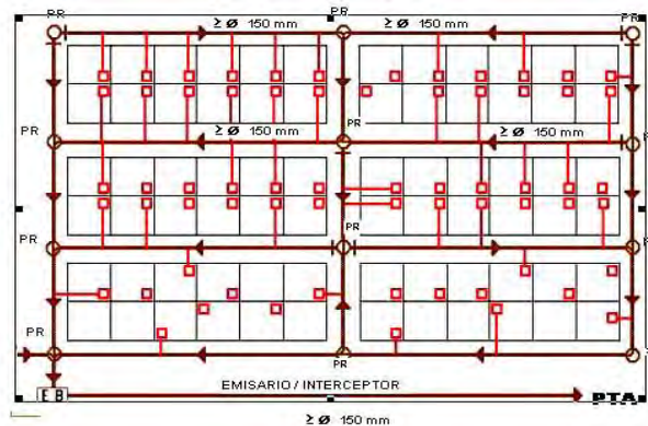
Figura 1. Componentes de un sistema de alcantarillado. Fuente: Rolim (1999).
