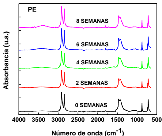
Figura 2. Espectros de FTIR de tinaco de PE expuesto a envejecimiento acelerado
