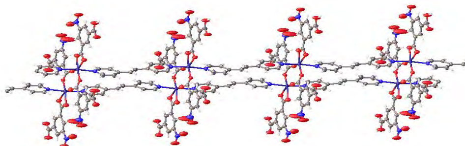
Figura 3. Vista de la estructura extendida del polímero mostrando el átomo de cobalto hexacoordinado, además de la presencia de los dos ligantes utilizados en la síntesis.
