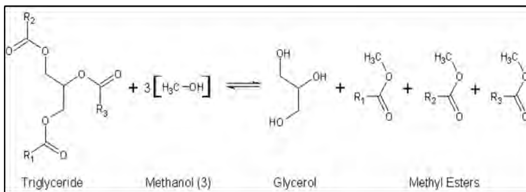
Figura 2. Reacción de transesterificación.
