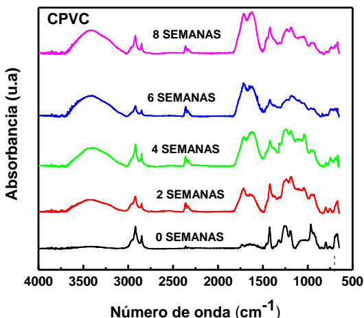
Figura 1.- Espectros de FTIR de tubería de CPVC expuesta a envejecimiento acelerado
