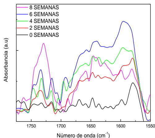
Figura 4. Espectros de FTIR de tinaco de PE expuesto a envejecimiento acelerado en la zona de carbonilos
