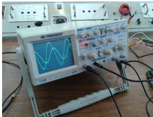
Figura 4. Defasamiento voltaje-corriente
