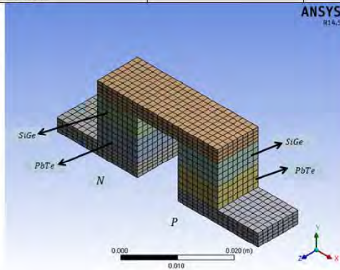
Figura 6. Esquema y resultados configuración 2
