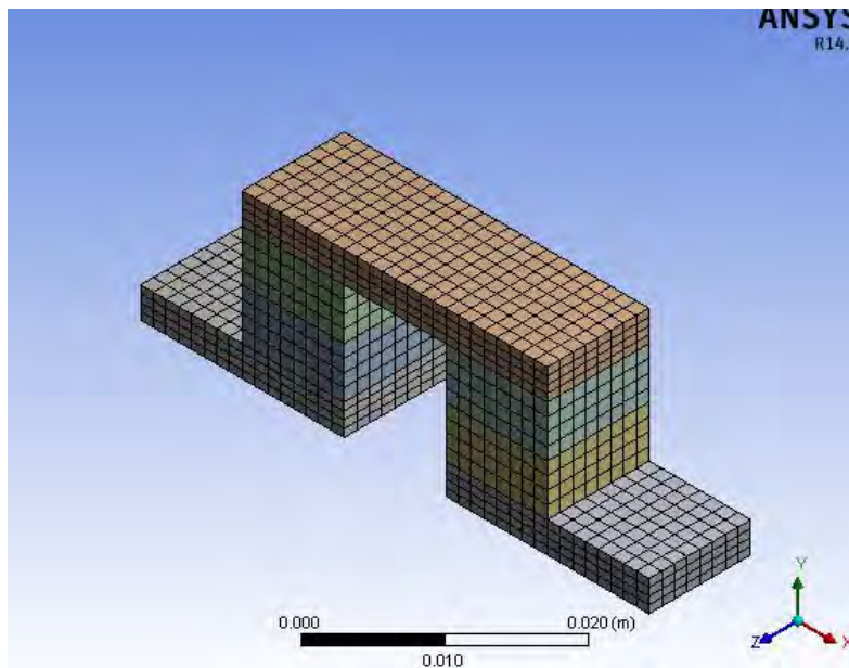
Figura 4. Mallado por Elemento Finito de un TEG Segmentado
