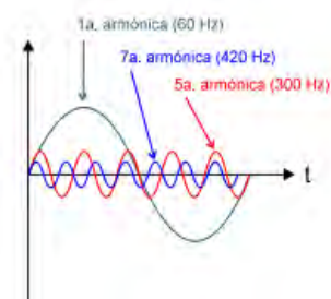
Figura 2. Componentes armónicos.
