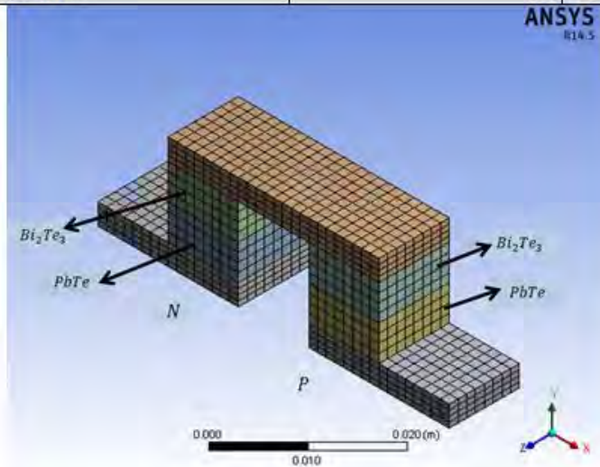
Figura 5. Esquema y resultados Configuración 1
