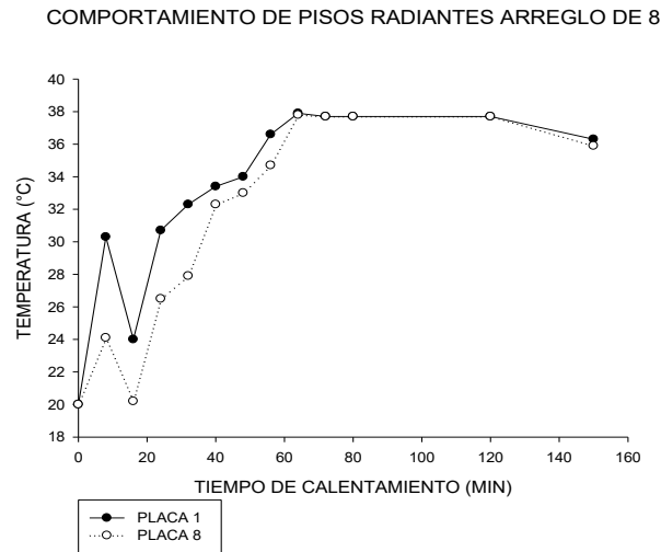
Figura 2. Gráfica de un arreglo de 8 pisos, cubriendo un ancho de 15.88 metros y un largo de 12.5 metros.
