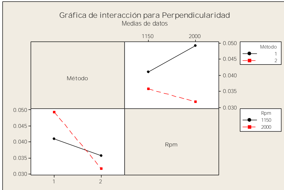
Figura 6. Gráfica de interacción para la perpendicularidad
