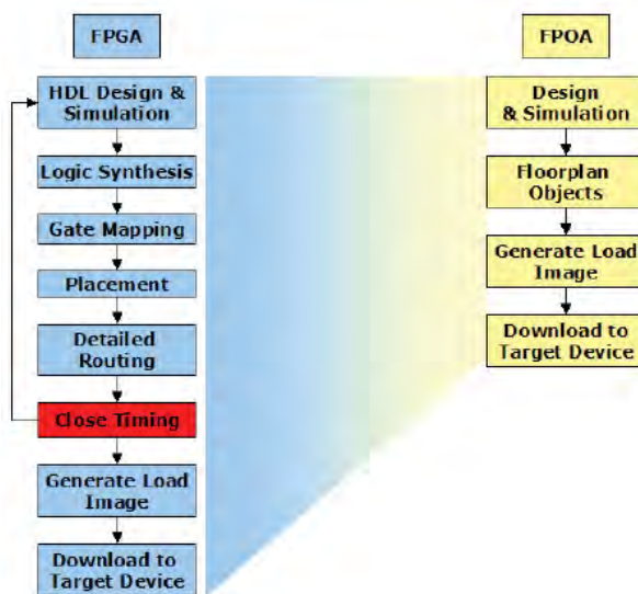
Figura 5. Comparación de flujo de diseño entre FPGA y FPOA.
