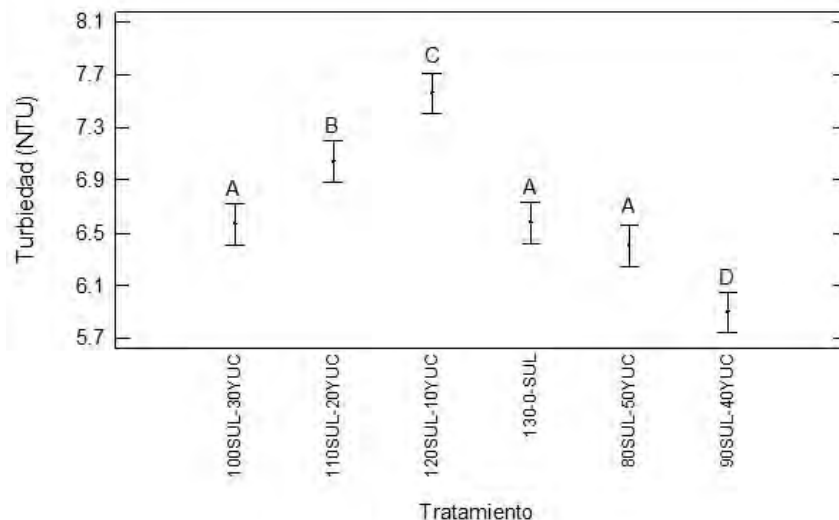
Figura 2. Valores promedios ( \pm ES) de la variable turbiedad de los tratamientos evaluados. Letras diferentes indican diferencias entre los tratamientos ( P < 0.05 ).
