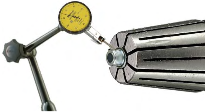
Figura 3. Medición del valor de perpendicularidad.
