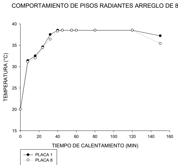
Figura 3. Gráfica de un arreglo de 8 pisos, cubriendo un ancho de 8 metros y un largo de 3.125 metros.
