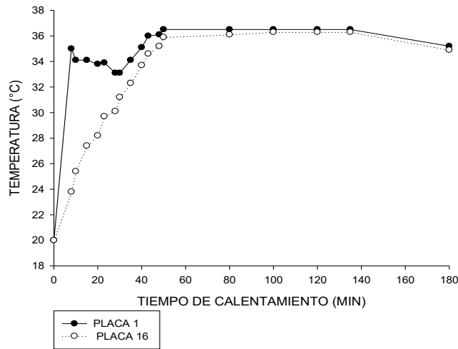
Figura 4. Gráfica de un arreglo de 16 pisos cubriendo un ancho de 15.88 metros y un largo de 12.5 metros.
