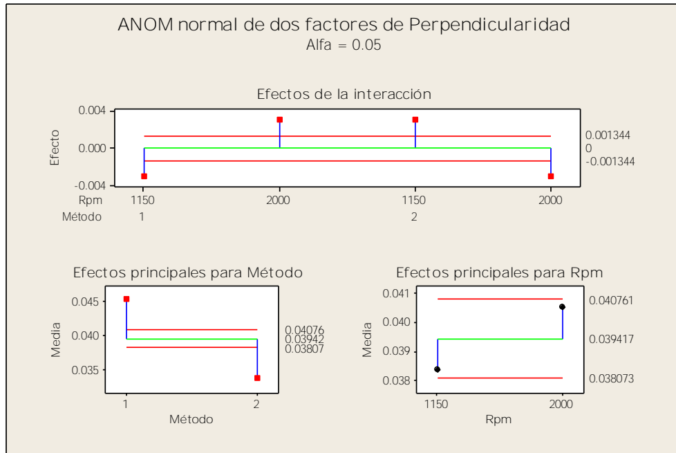
Figura 4. Análisis de medias para la perpendicularidad.
