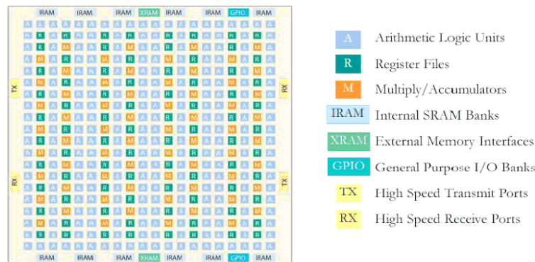
Figura 2. Red de FPOA [MathStar].
