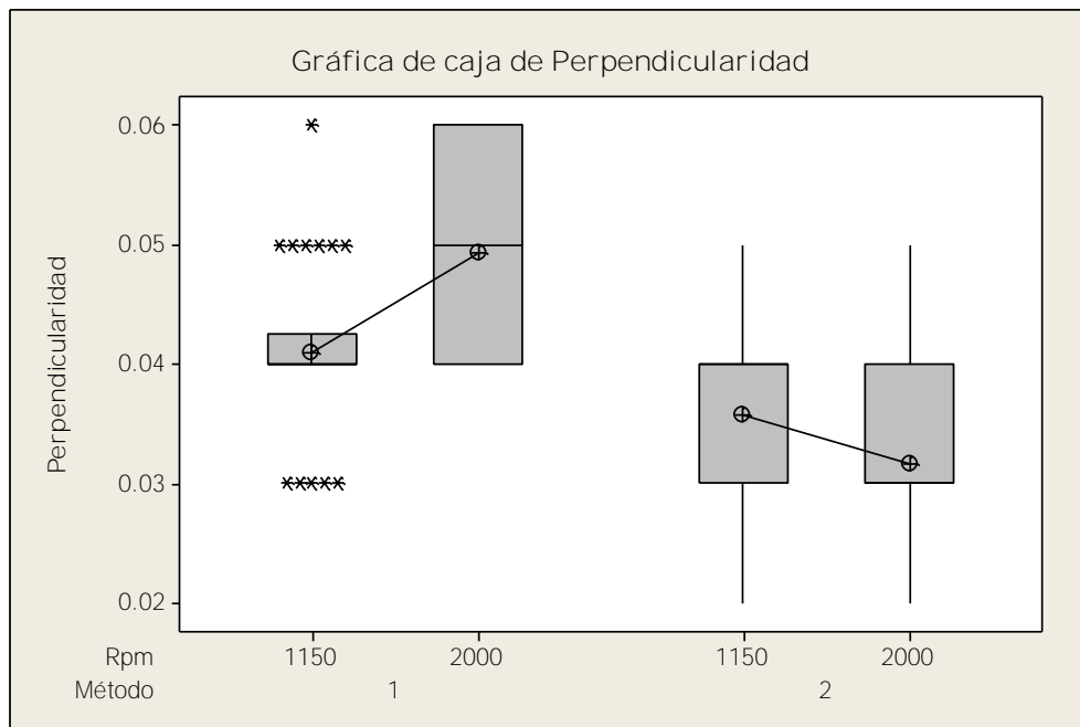
Figura 5. Gráfica de cajas para la perpendicularidad.
