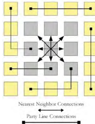
Figura 4. Los dos tipos de conexión para un FPOA [MathStar].
