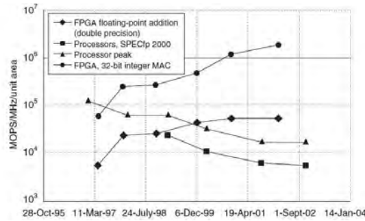
Figura 1. Densidad computacional de FPGAs y procesadores Intel. (Chang C, et. al., 2005)
