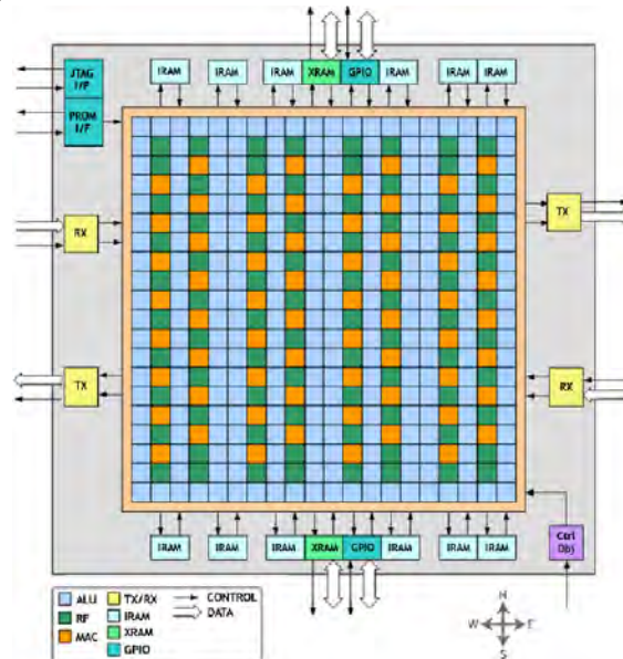
Figura 3. Muestra las dos superficies generales de un FPOA [MathStar].
