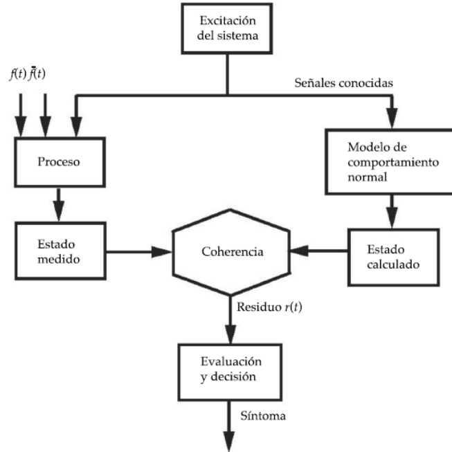
Figura 1 Principio de la obtención del residuo r(t) y síntoma de fallas donde f(t) son las fallas de interés y \tilde{f}(t) denota perturbaciones y ruido.
