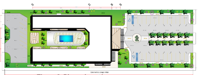
Figura 8. Planta de conjunto
