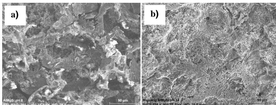
Figura 5. Micrografías de la superficie de probetas de Al-Mg-Si expuestas en agua de mar sintética: a) pH 8 b) pH 14, ajustados con NaOH.
