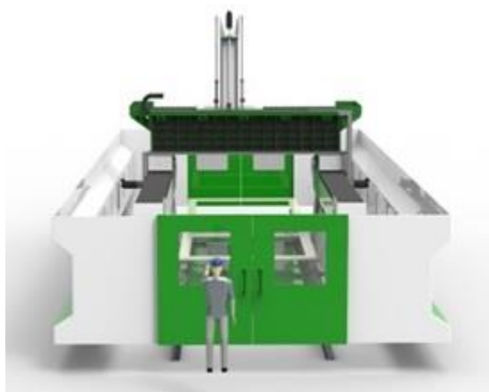
Figura 2. Representación de vista frontal de máquina de cinco ejes.
