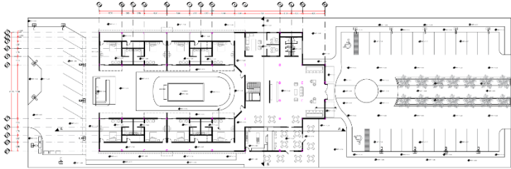
Figura 5. Planta arquitectónica primer nivel
