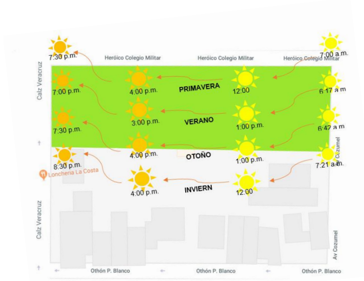
Figura 2. Representación de asoleamiento en el terreno.
