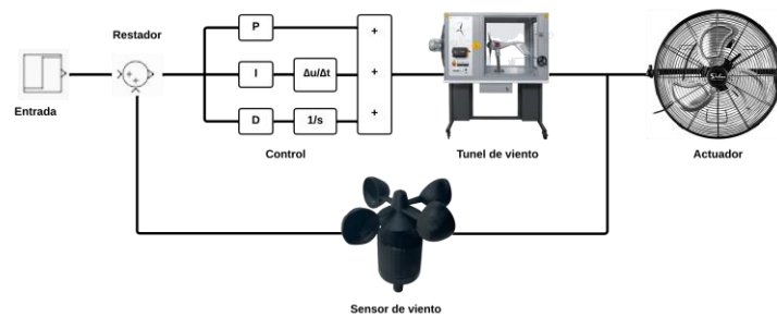
Figura 3. Diagrama a bloques del sistema de control.
