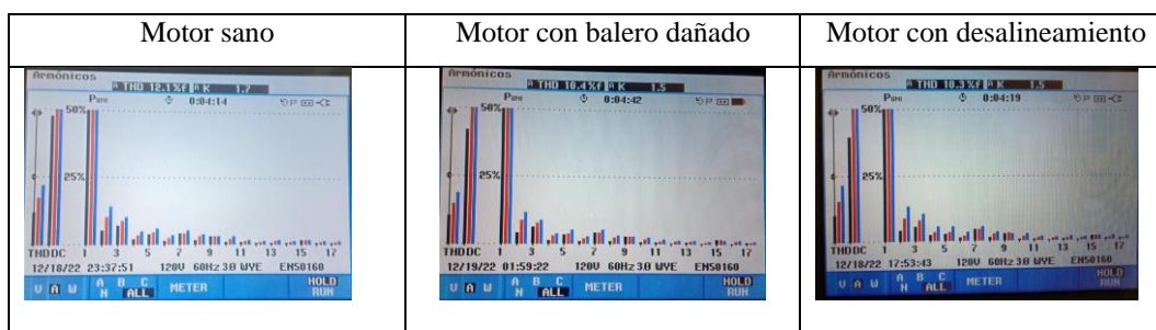
Cuadro 4. Señales de armónicos en corriente eléctrica.
