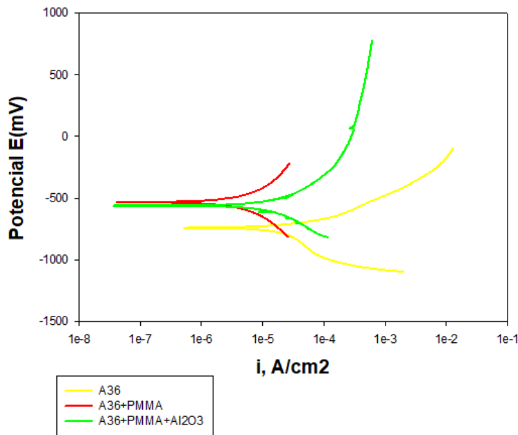
Figura 6. Curvas Rp de los tres sistemas bajo tres condiciones diferentes.
