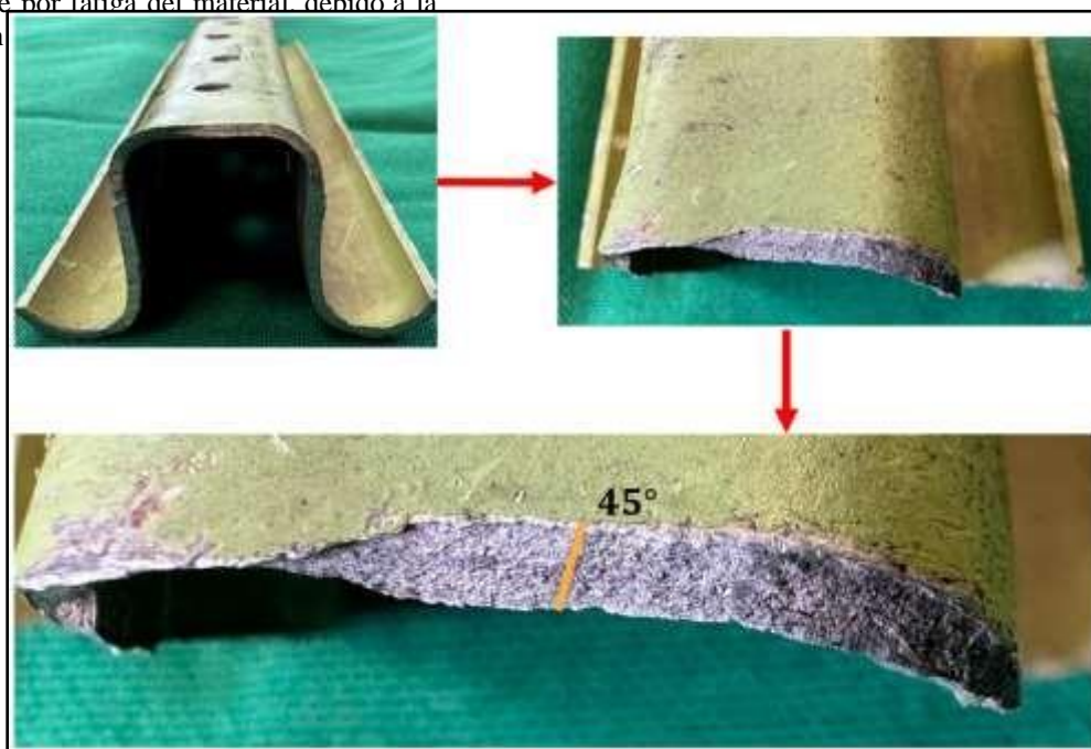
Figura 6. Acercamiento en zona de ruptura.
