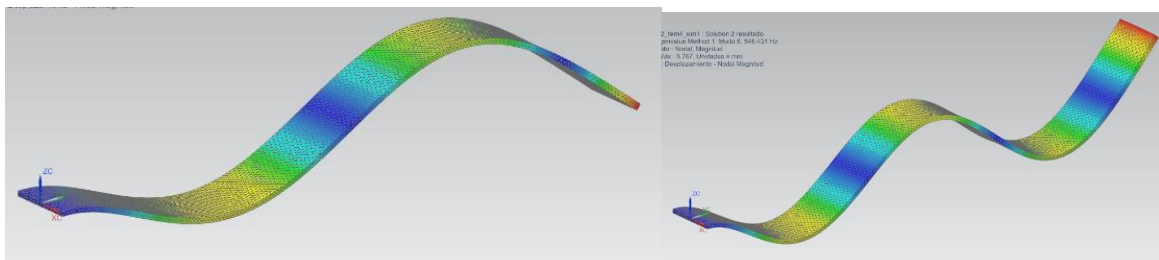
Figura 6. Tercer y cuarto modo de vibración.
