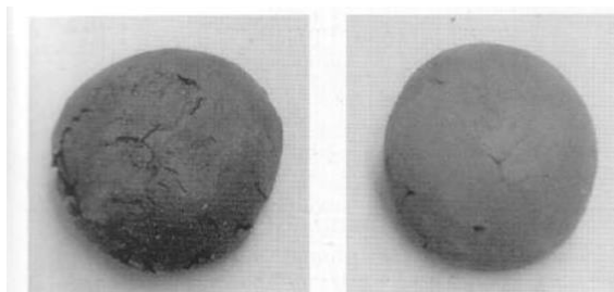
Ilustración 8.-Ensayo de caída de bola. Sirve para demostrar diferentes cohesividades. Fuente: Minke, G. (2005). Manual de construcción
