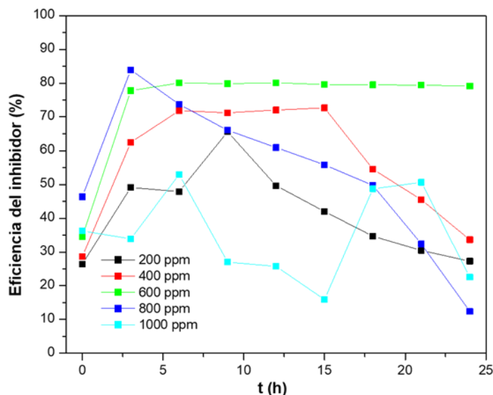
Figura 3. Curvas de eficiencias del inhibidor obtenidas sobre el acero 1018 sin y con inhibidor. }
