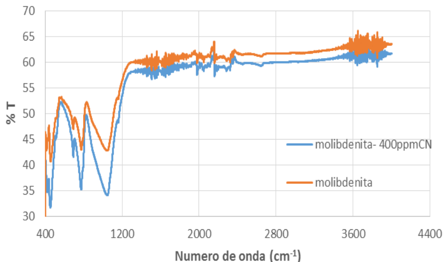
Figura 8. Espectro Infrarrojo de la molibdenita antes y después del proceso de cianuración
