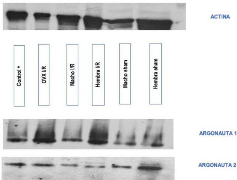
Figura 1- Resultado experimental de la detección de proteínas ArgonAUTAs. Western blot de las proteínas ArgonAUTAs (1 y 2) en las diferentes condiciones experimentales descritas en cada carril. Se utilizó como control positivo de expresión un lisado celular de la línea Caco.
