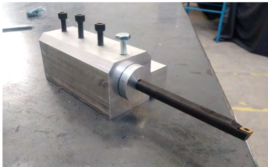
Figura.26 Pieza Terminada.
