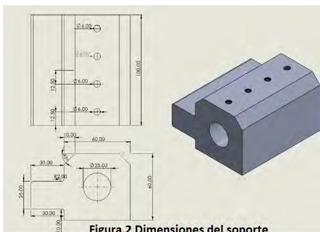
Figura.2 Dimensiones del soporte
