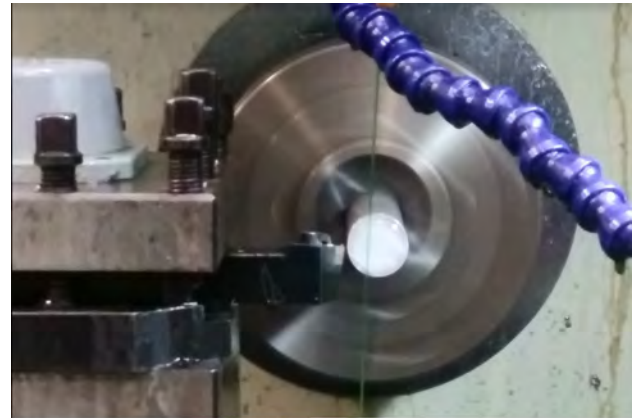
Figura.17 Careado del cilindro
