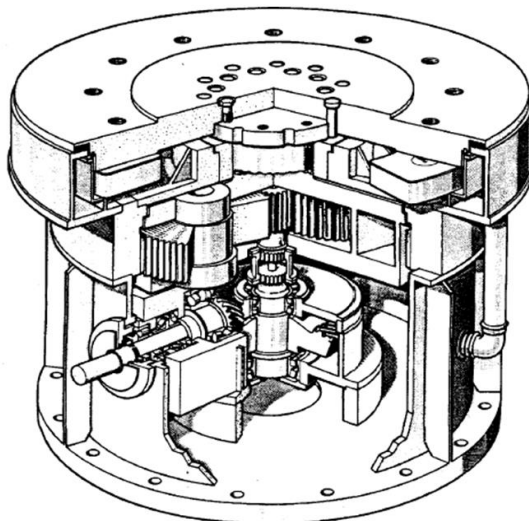
Figura 2. Reductor MAAG Modelo WPU-161E.
