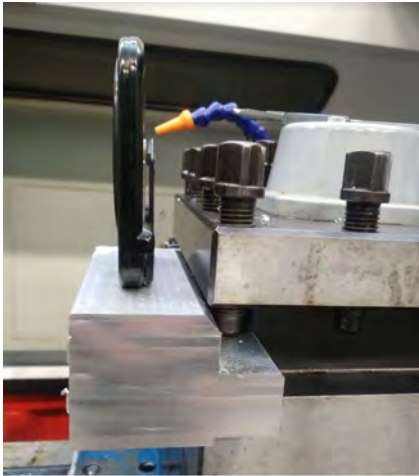
Figura.9 Pieza colocada en el torno CNC
