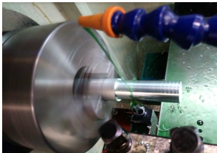
Figura.18 Desbaste de Cilindro.
