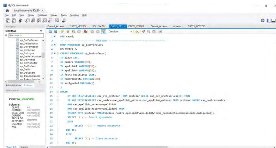
Figura 1. Procedimiento almacenado (sp_InsProfesor) para validar el registro de un docente
