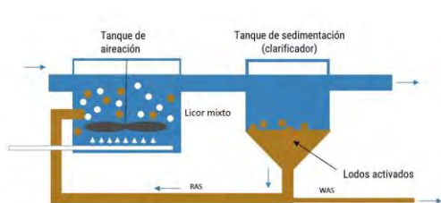
Figura 2: Lodos Activados
