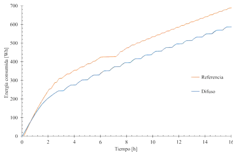
Figura 5. Consumo de energía del refrigerador.
