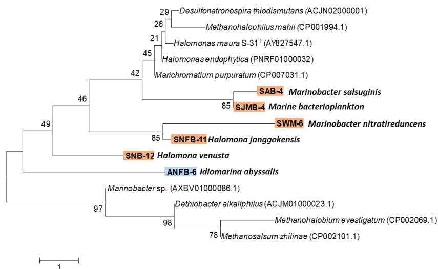
Figura 3. Árbol filogenético Neighbour Joining del gen nifH de las cepas bacterianas halófilas.
