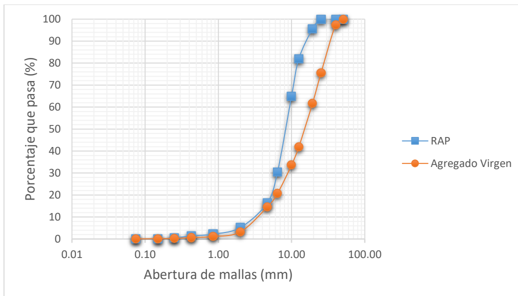
Figura 1. Curvas granulométricas de los agregados vírgenes y RAP
