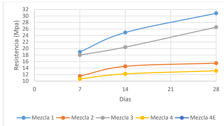
Figura 2. Resistencia a la compresión simple de las mezclas a diferentes días.
