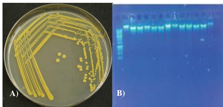
Figura 1. A) Cepa pura aislada. B) Electroforesis de ADN genómico de cada cepa.
