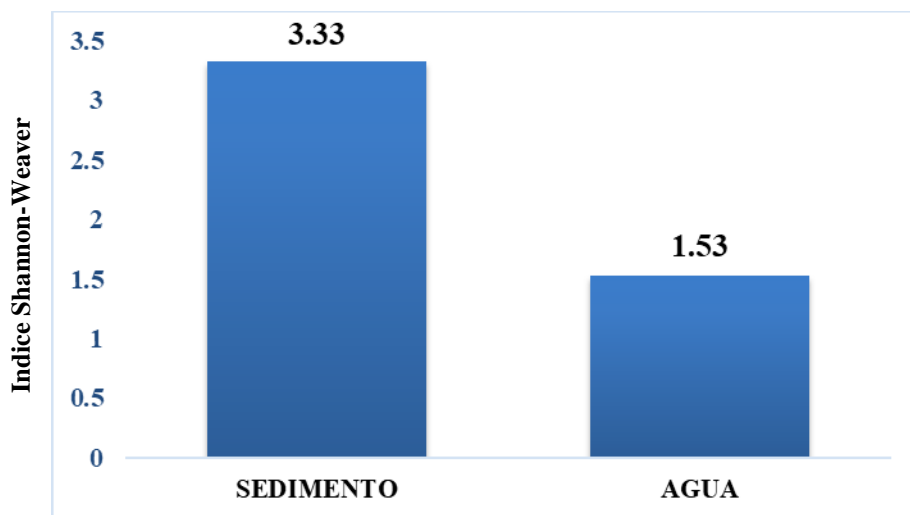
Figura 2. Índice de diversidad (H) de especies de bacterias halófilas fijadoras de nitrógeno
