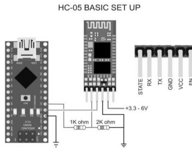
Figura 3. Módulo bluetooth.
