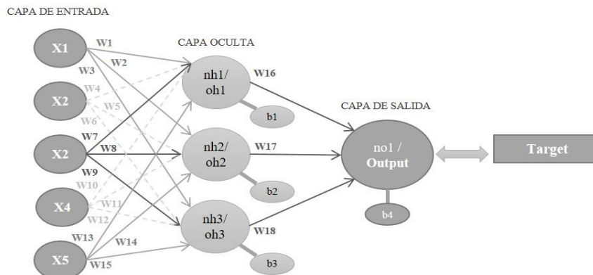
Figura 2. Arquitectura de la Red 5-3-1
