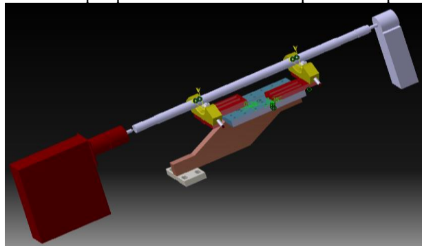
Figura 4. Simulación del ajuste de semieje (vista 3D).
