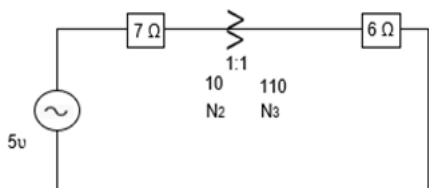
Figura 4. Circuito eléctrico simplificado con valores en ohms del sistema de prueba
