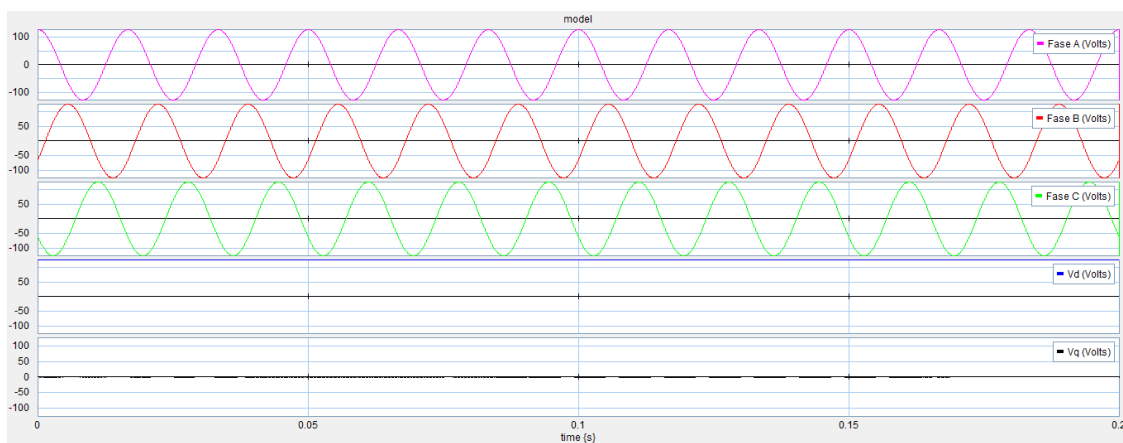
Figura 3.0 Transformación de Park en 20Sim.
