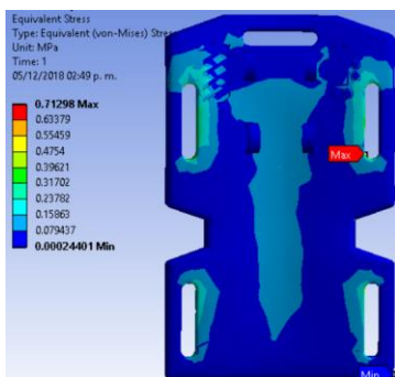
Figura 13. Teoría de fallo: Estrés equivalente de Von Mises
