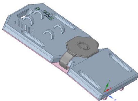
Figura 10. Diseño final del dispositivo reanimador cardíaco
