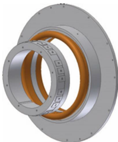
Figura 1.0 Generador de imanes permanentes de neodimio-cobalto.
