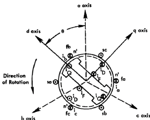
Figura 2.0 Representación pictórica del marco de referencia dq0.
