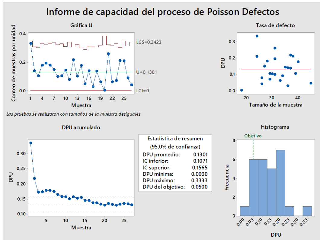
Figura 4 Informe de capacidad del proceso
