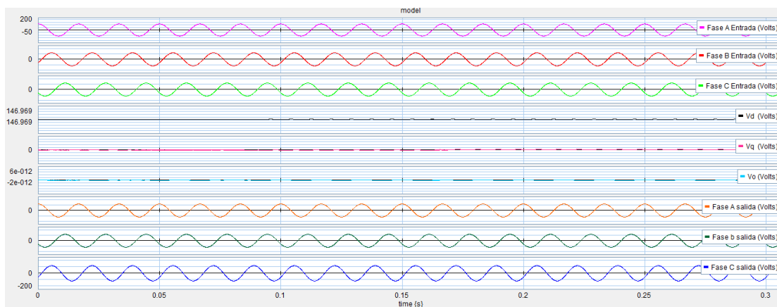
Figura 4.0 Transformación inversa de Park en 20Sim.
