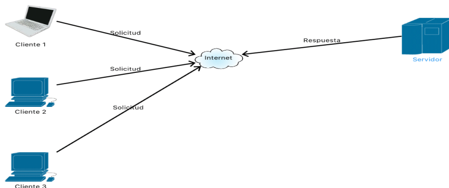
Figura 3. Arquitectura cliente-servidor.
