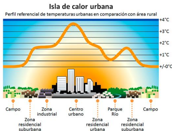
Figura 1 muestra el perfil de referencia de una isla de calor.
