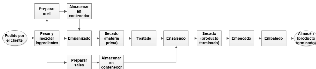
Fig. 1. Mapa de flujo de proceso de nivel 1 producción de cacahuates tipo japones
