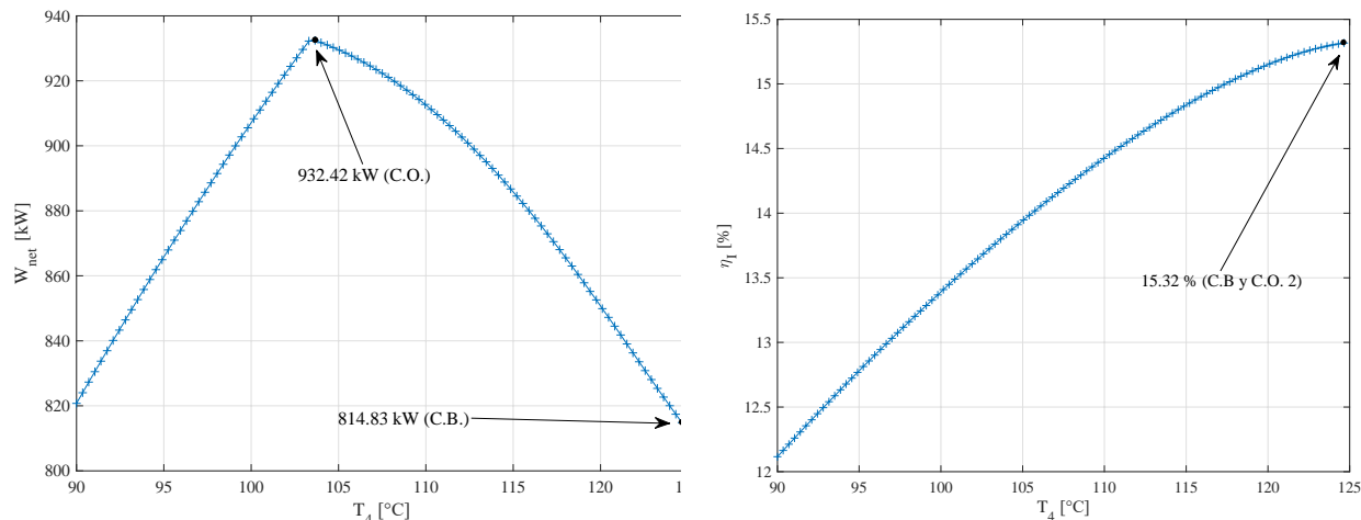
Figura 3. Variación del trabajo neto (izquierda) y la eficiencia energética (derecha) en el ORC.
