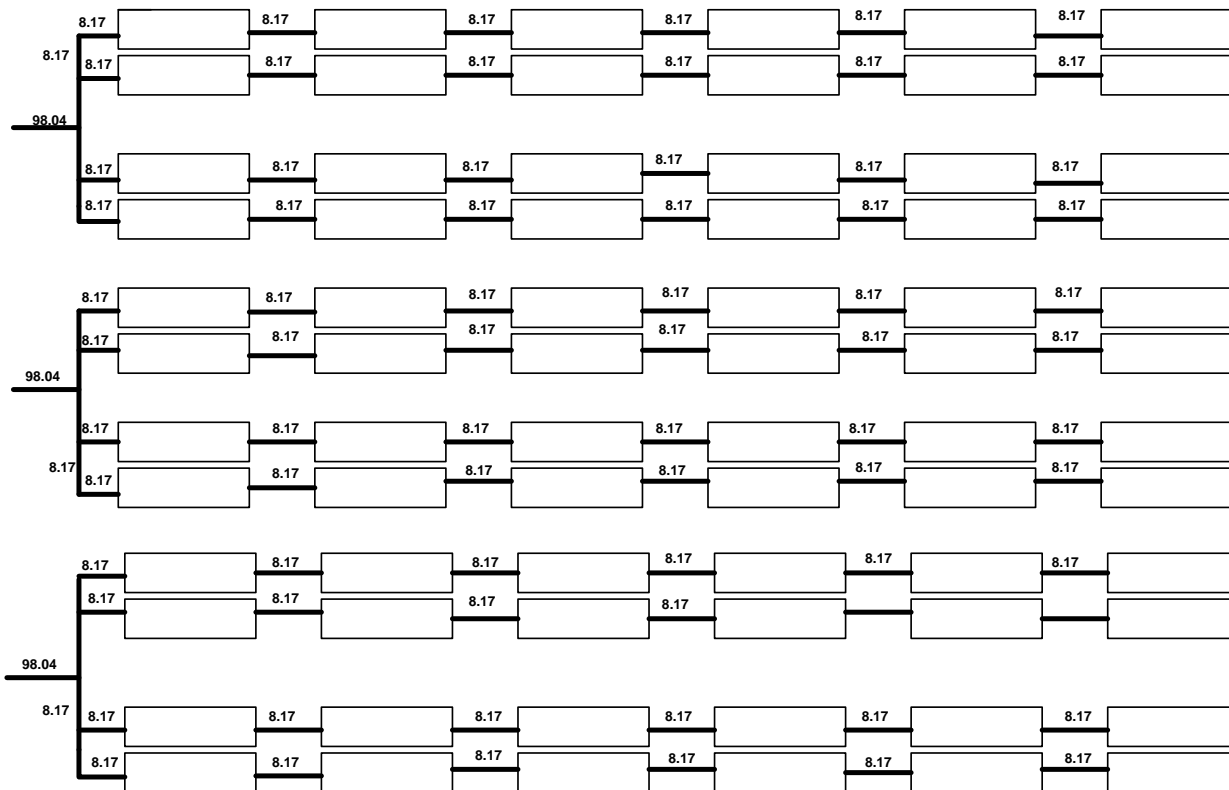
Figura 7 Conexión de Celdas fotovoltaicas
