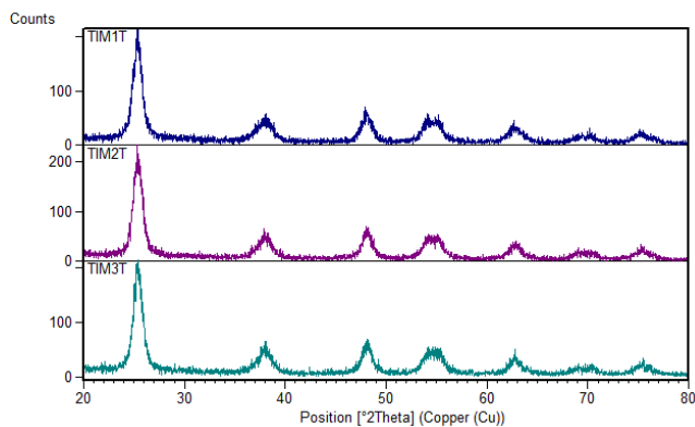
Figura 4. Espectros de DRX muestras TIM1T, TIM2T Y TIM3T.
