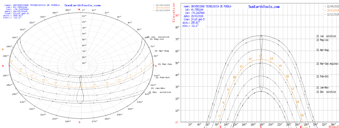
Figura 2. Movimiento del sol relativo a la ubicación y Horas de sol efectivas en el lugar
