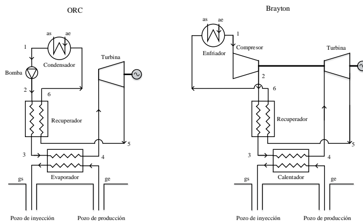
Figura 1. Configuración esquemática de los sistemas.
