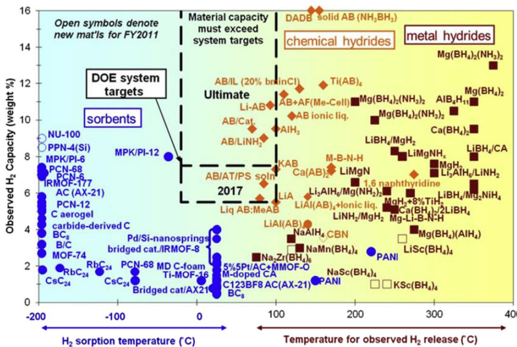
Figura 1. Capacidad de almacenamiento de Hidrógeno de materiales comúnmente empleados con respecto a la temperatura de operación. (S. Satyapal, U.S. Department of Energy.)
