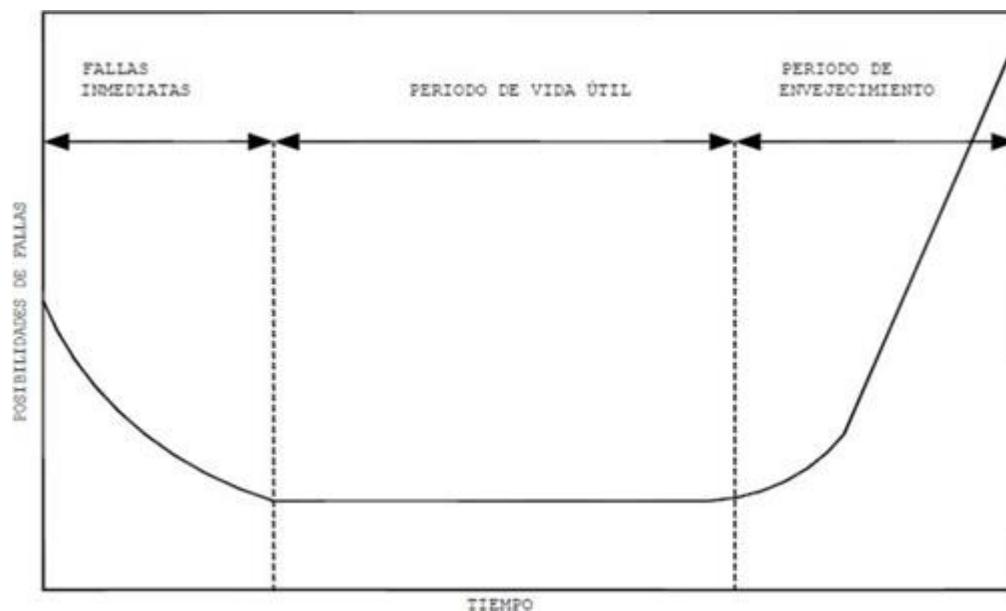
Figura 2 Curva de vida útil de un transformador de potencia.
