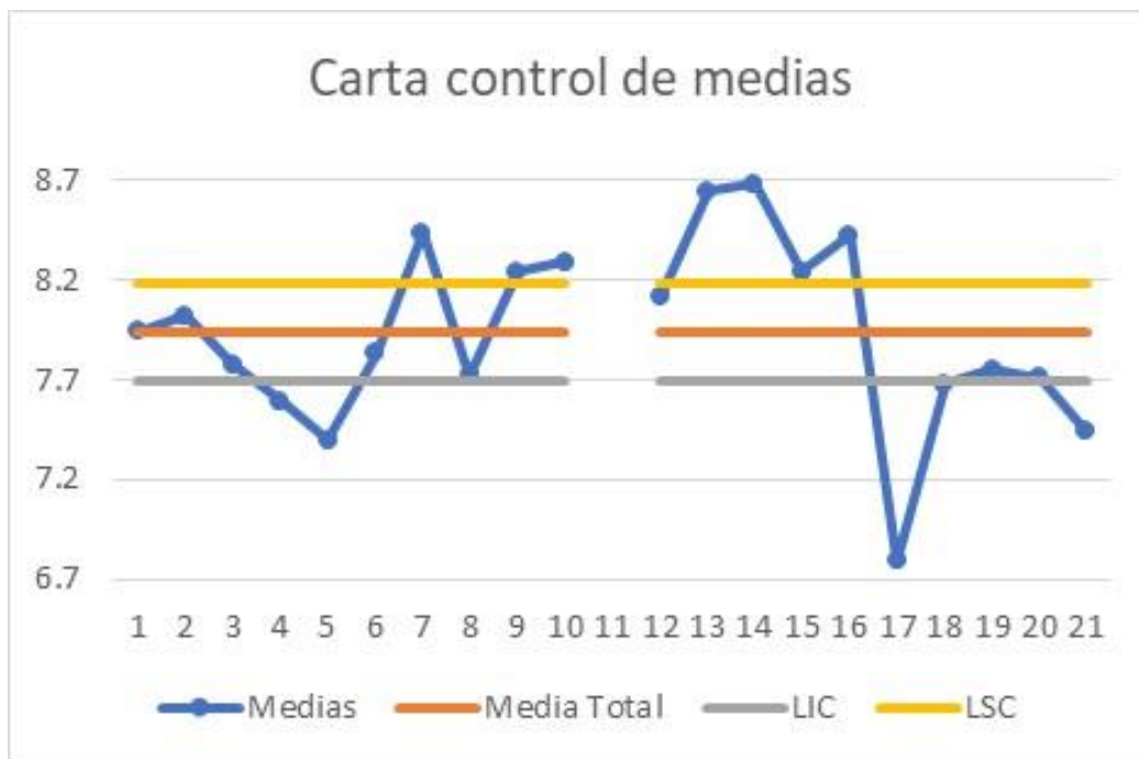
Gráfica 3. Carta de control de medias
