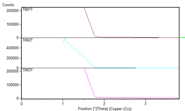
Figura 5. Espectros de DRX a ángulo bajo de las muestras TIM1T, TIM2T Y TIM3T
