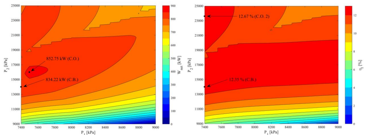
Figura 4. Variación del trabajo neto (izquierda) y la eficiencia energética (derecha) en el ciclo Brayton.
