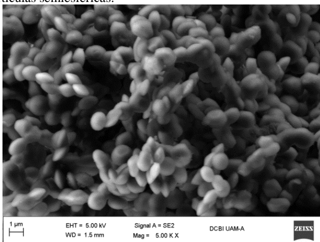
Figura 6. Micrografía SEM de las muestras SiO 2 .
