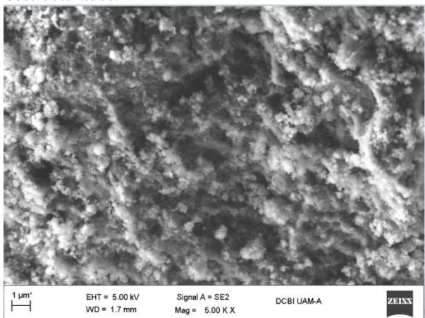
Figura 8. Micrografía SEM de las muestras Al 2 O 3 .
