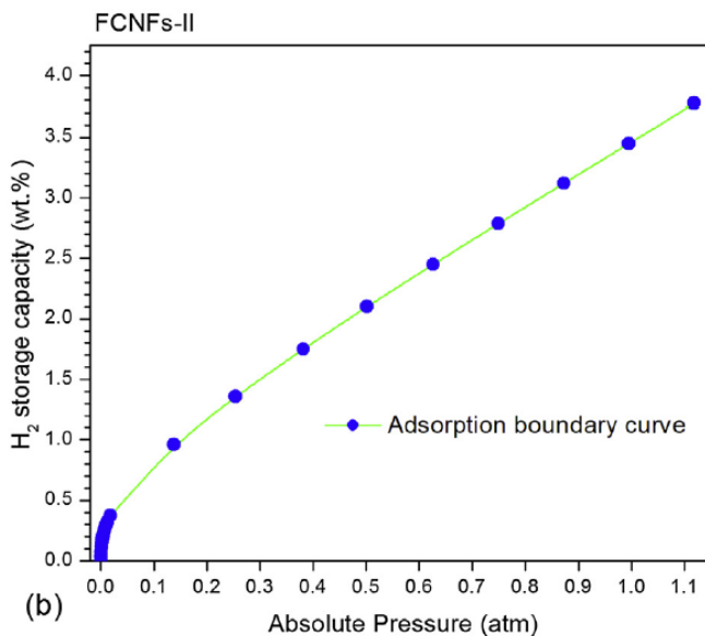
Figura 2. Gráfica de la capacidad de almacenamiento de hidrógeno de un material poroso funcionalizado (Felix Galindo Hernandez, 2014).
