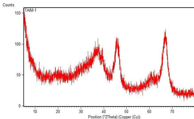
Figura 4. Espectros de DRX de la muestra TAIM-1.
