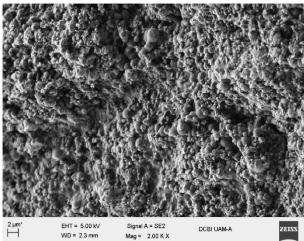
Figura 7. Micrografía SEM de las muestras TiO 2 . 3. Al 2 O 3
