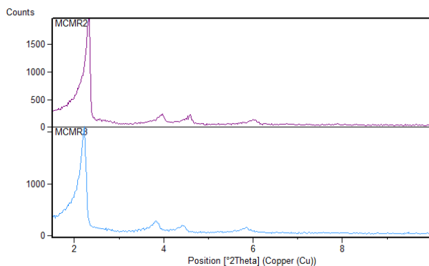
Figura 3. Espectros de DRX muestras MCMR2 y MCMR3
