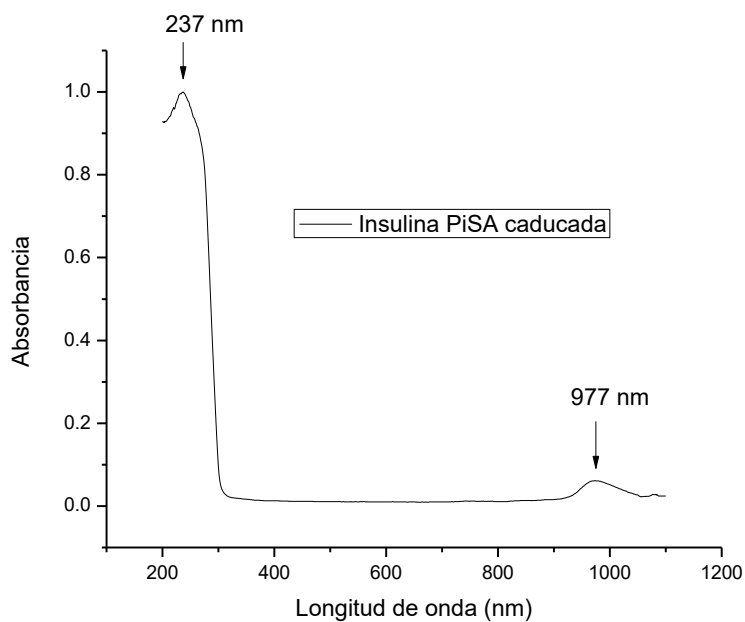
Figura 2. Forma de línea UV-Vis de la molécula de la insulina de acción rápida caducada
