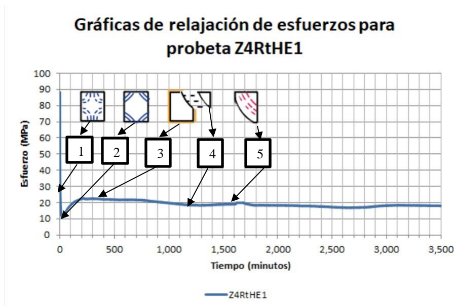
figura 9 gráfica de relajación y esquematización del mecanismo cíclico para probeta ensayada a 40 °C, a una rapidez de deformación de 8.33 \times 10^{-3} \text{s}^{-1} y una deformación de ensayo del 4%.
