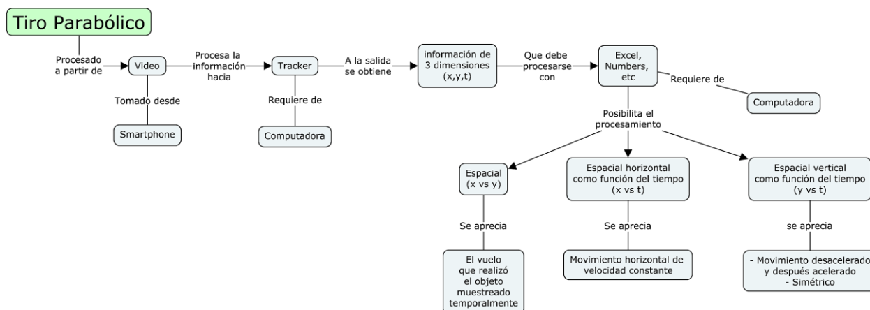
Figura 2. Esquema de procesamiento del tiro parabólico con ayuda de smartphone y computadora.
