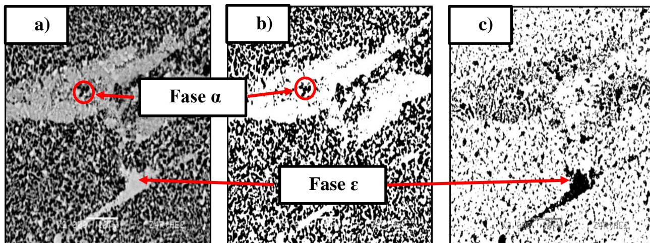
Figura 5 a) metalografía original de la aleación Zn-22%Al-4%Ag, b) imagen procesada y reconocimiento de la fase \alpha , c) imagen procesada y reconocimiento de la fase \epsilon
