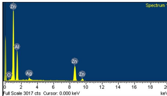
Figura 2 Espectro EDS de la aleación Zn-22%Al-4%Ag
