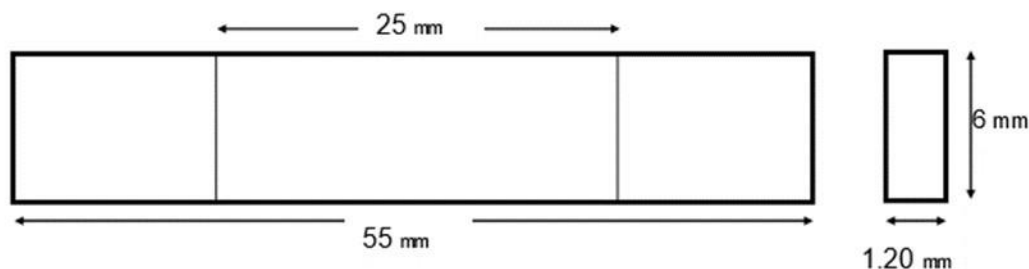
Figura 3 Diseño de probetas para ensayos de relajación de esfuerzos.
