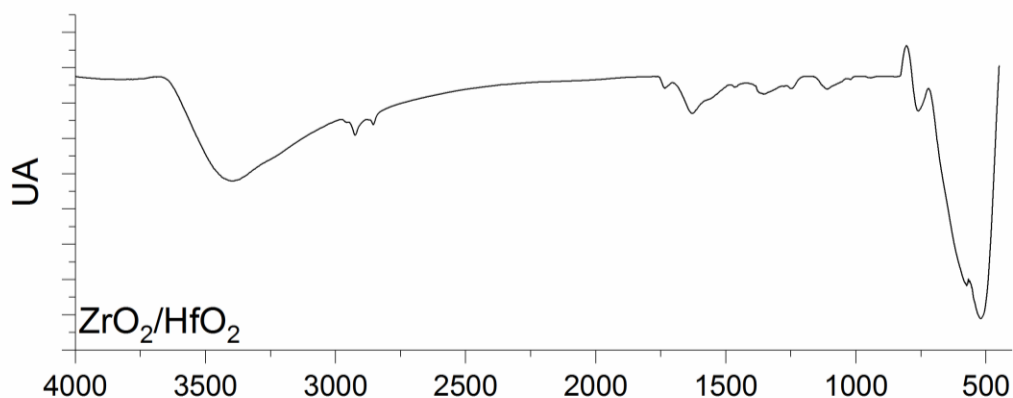
Figura 1 Espectros FTIR de circonia modificada con hafnio
