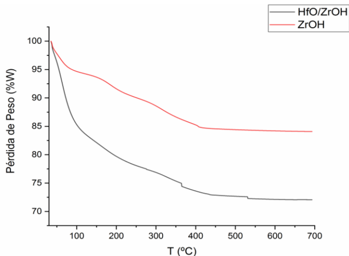
Figura 2. Análisis térmico-gravimétrico TGA de los hidróxidos precursores
