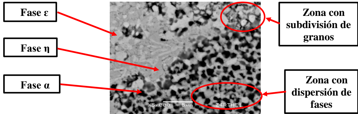
Figura 1 Zn-22%Al-4%Ag ensayada a 40 °C con una rapidez de deformación de 8.333 \times 10^{-3} \text{s}^{-1} y una deformación de 4%
