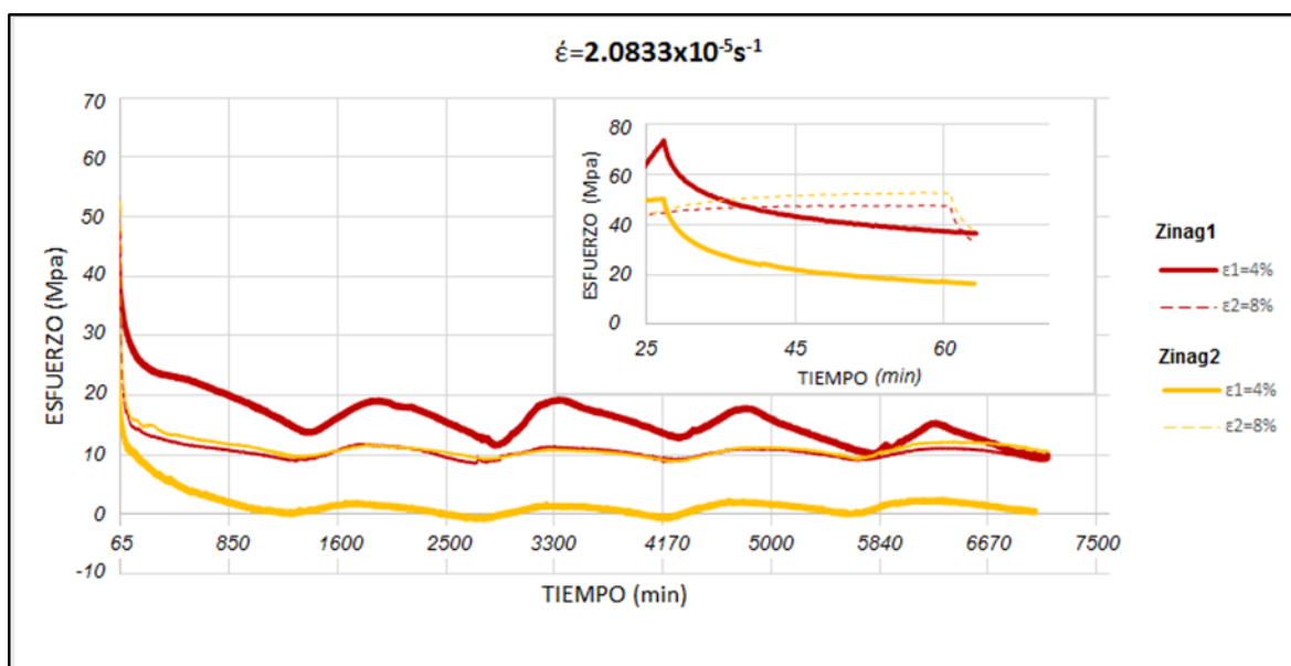
Figura 2 curvas de relajación ensayadas a una rapidez de deformación de 2.0833 \times 10^{-5} s^{-1} en aleaciones Zinag con 1 y 2% en peso de Ag a deformaciones de 4 y 8%.
