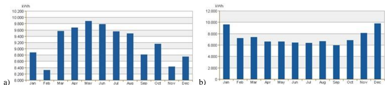
Figura 4. Consumo eléctrico mensual, a) equipos convencionales, b) bomba de calor geotérmica.
