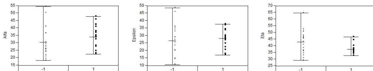
Figura 7 gráficas de dispersión para las deformaciones -1 = 4% y 1 = 8%; a) fase \alpha , b) fase \epsilon , c) fase \eta
