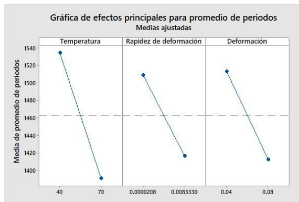
figura 6 gráfica de efectos principales para promedio de periodo
