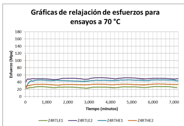
figura 4 curvas de relajación ensayadas a 70°C
