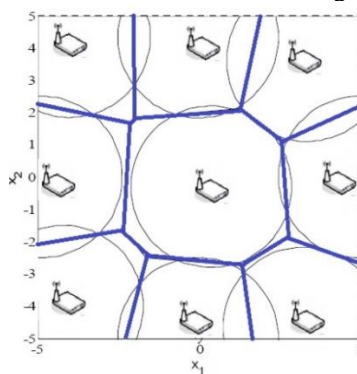
Figura 6. Diagramas de Voronoi cubriendo un área
