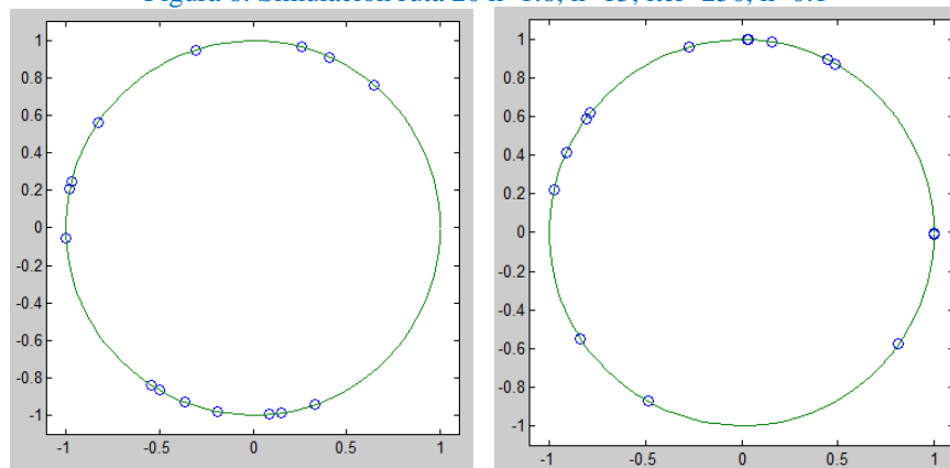
Figura 9. Simulación ruta 20 k=0.1 , n=15 , iter=250 , h=0.1
