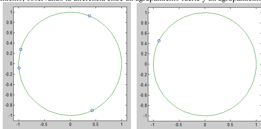
Figura 6. Simulación ruta penal k=1.8 , n=4 , iter=250 , h=0.1
