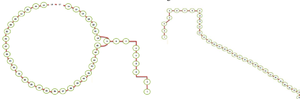
Figura 3. Red compleja de ruta 20 (izquierda) y ruta 41 (derecha)
