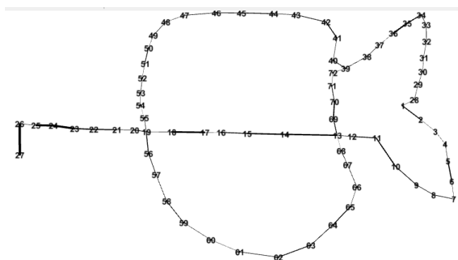
Figura 5. Red compleja de las dos rutas.
