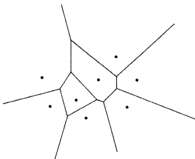
Figura 5. Diagrama de Voronoi para ocho puntos en el plano
