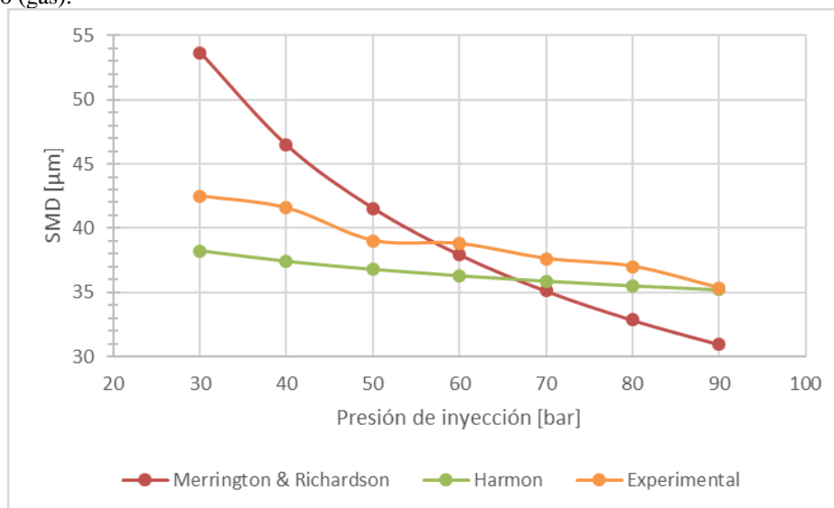
Figura 4. Curvas del diámetro medio de Sauter en función de la presión de inyección.
