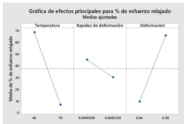
figura 7 gráfica de efectos principales para el porcentaje del esfuerzo relajado
