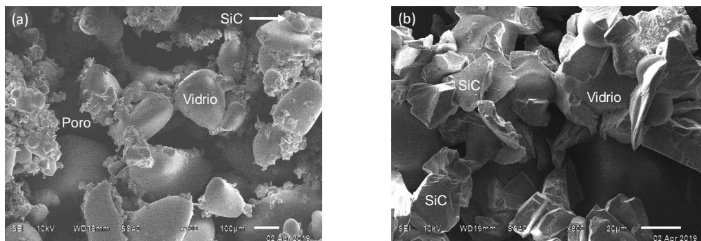
Figura 2. Imágenes de Microscopía Electrónica de Barrido de la muestra tratada a 775°C con 20 min de permanencia. (a) 100x, (b) 800x.
