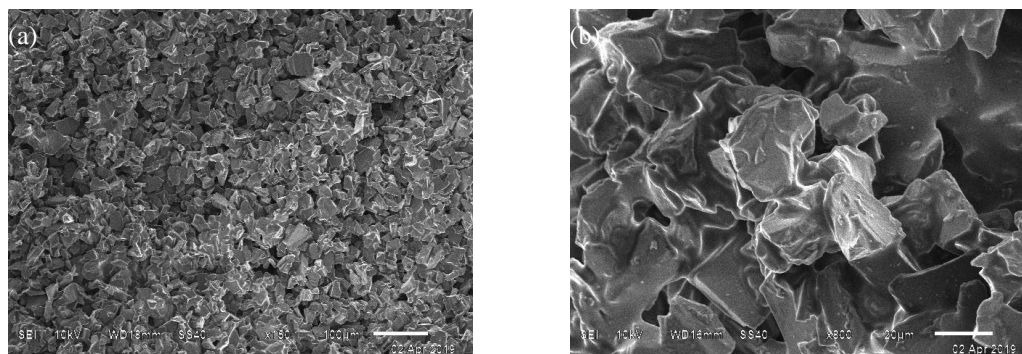
Figura 3. Imágenes de Microscopía Electrónica de Barrido de la muestra tratada a 800°C con 30 minutos de permanencia. (a) 100x, (b) 800x
