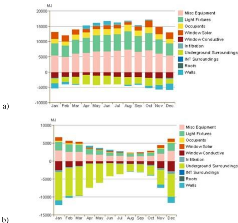
Figura 3. Acumulativo mensual de carga térmica, a) enfriamiento, b) calefacción.
