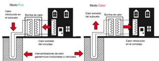
Figura 1. Esquema de una bomba de calor con intercambiadores de calor geotérmicos.
