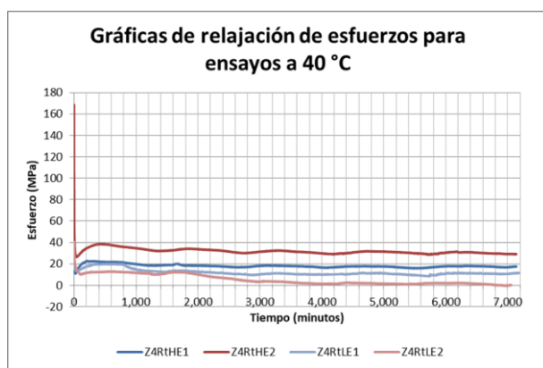
figura 3 curvas de relajación ensayadas a 40°C
