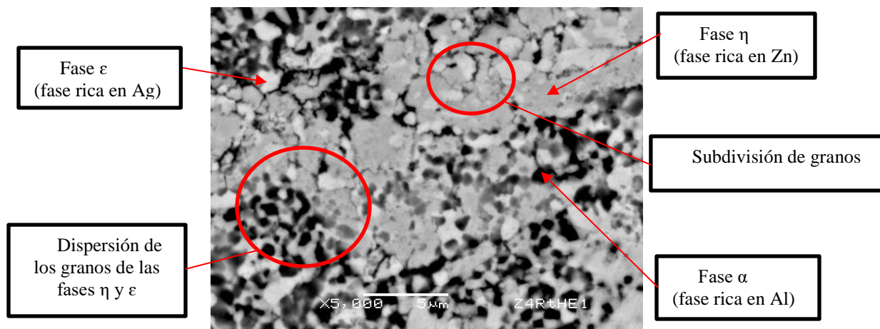
figura 8 metalografía para probeta Z4RtHE1
