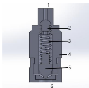
Figura 1. Diagrama de la construcción de la esprea. donde 1 es la entrada del líquido, 2 el embolo superior, 4 la carcasa de la esprea, 5 el embolo inferior, 6 el orificio de salida del chorro.
