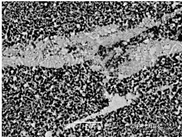
Figura 4 Metalografía de probeta ensayada a 40°C con deformación al 8%
