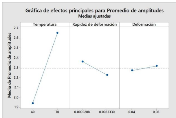
figura 5 gráfica de efectos principales para promedio de amplitudes
