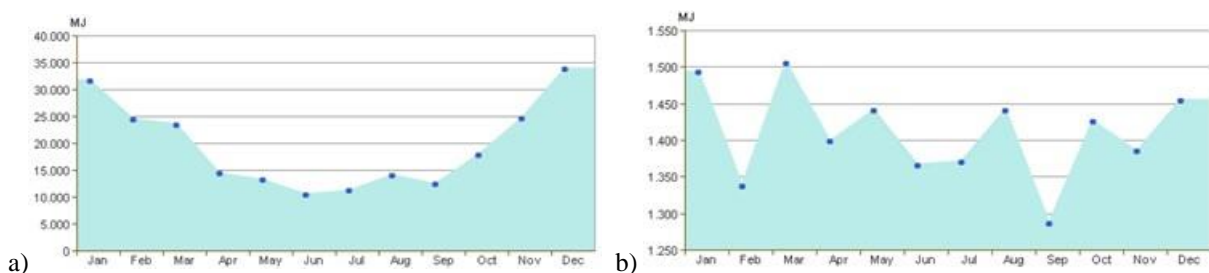
Figura 5. Consumo de combustible mensual, a) equipos convencionales, b) bomba de calor geotérmica.
