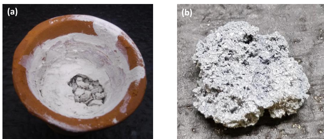
Figura 1. Imágenes de cerámicos tratados térmicamente a 775^\circ\text{C} . (a) Nitruro de silicio, (b) Carburo de silicio
