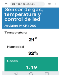
Figura 4. Datos generados por el arduino.
