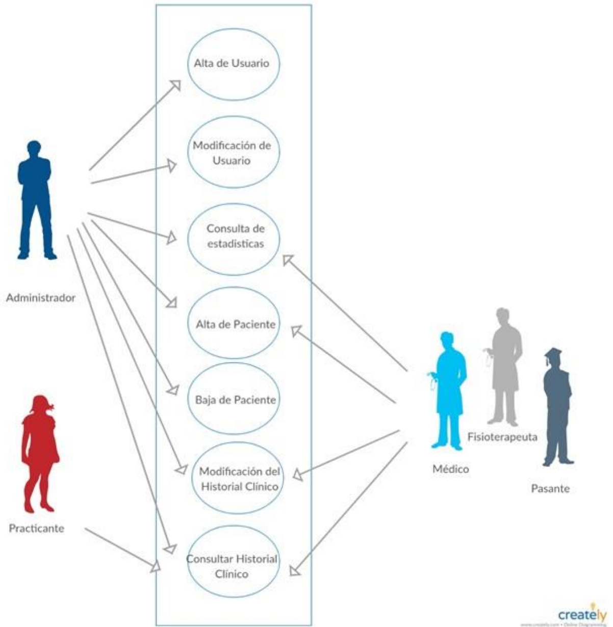
Figura 2. Caso de Uso UML, Actores que intervienen en el sistema
