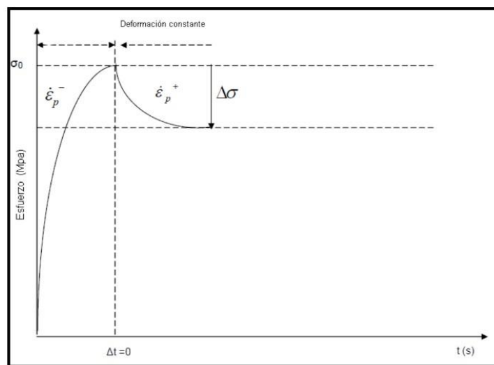
Figura 1 ejemplo de curva de relajación de esfuerzos
