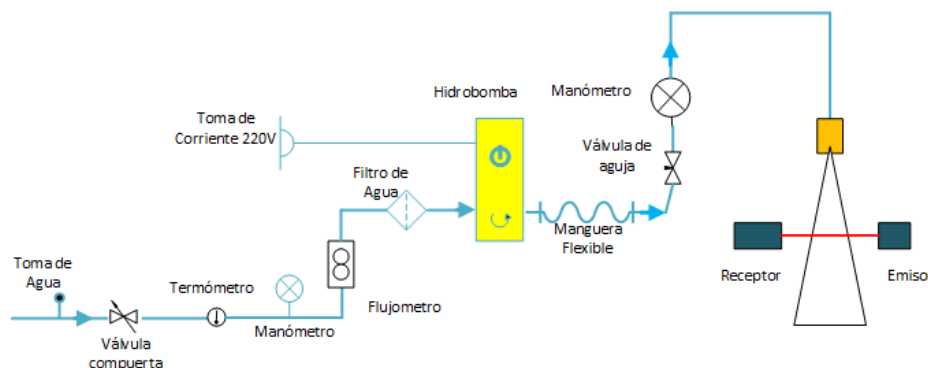
Figura 2. Diagrama de la instalación experimental.
