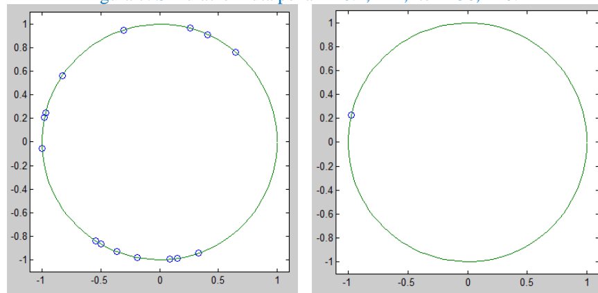
Figura 8. Simulación ruta 20 k=1.8 , n=15 , iter=250 , h=0.1
