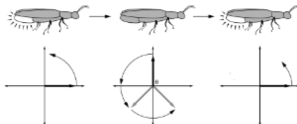
Figura. 1 Sincronización de luciérnagas.
