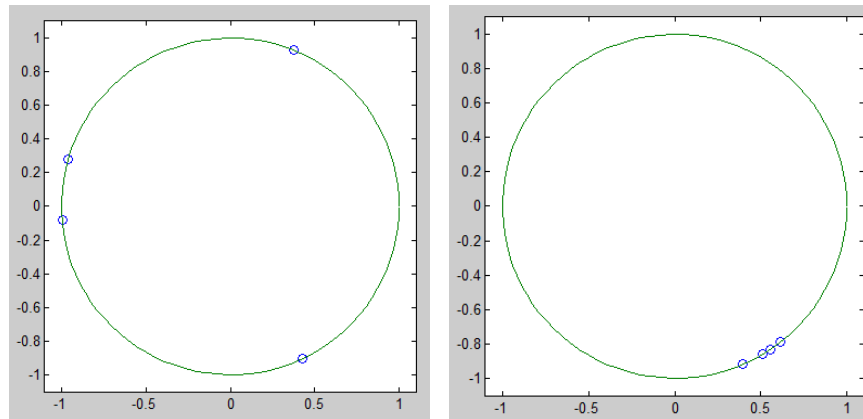
Figura 7. Simulación ruta penal k=0.1 , n=4 , iter=250 , h=0.1
