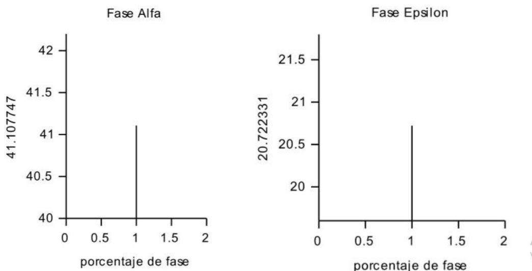
Figura 6 Cuantificaciones de las fases presentes en la metalografía
