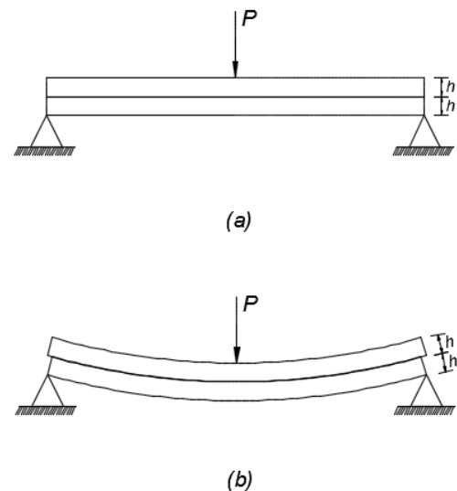
Figura 2- Flexión de dos barras independientes sobrepuestas.
