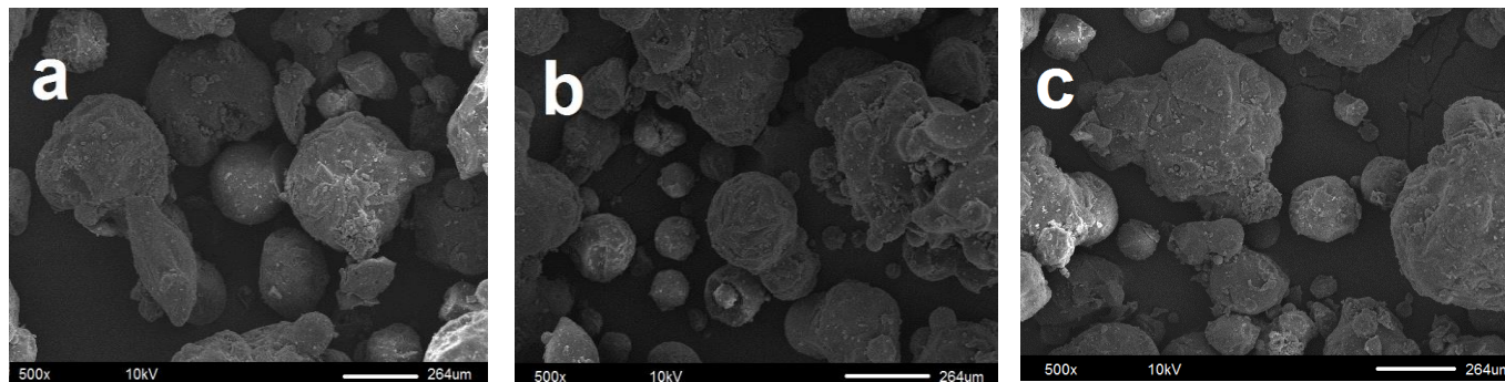
Figura 3. Microscopía electrónica de barrido de los polvos obtenidos a diferente temperatura. a, 70°C. b 80 °C. c, 90°C.
