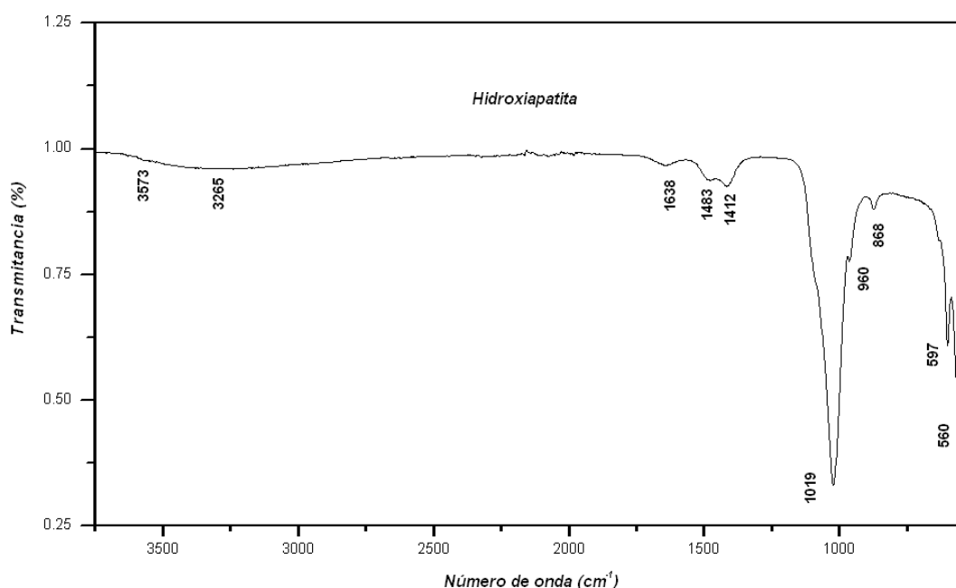
Figura 3. Espectro de infrarrojo de Hidroxiapatita (HA)
