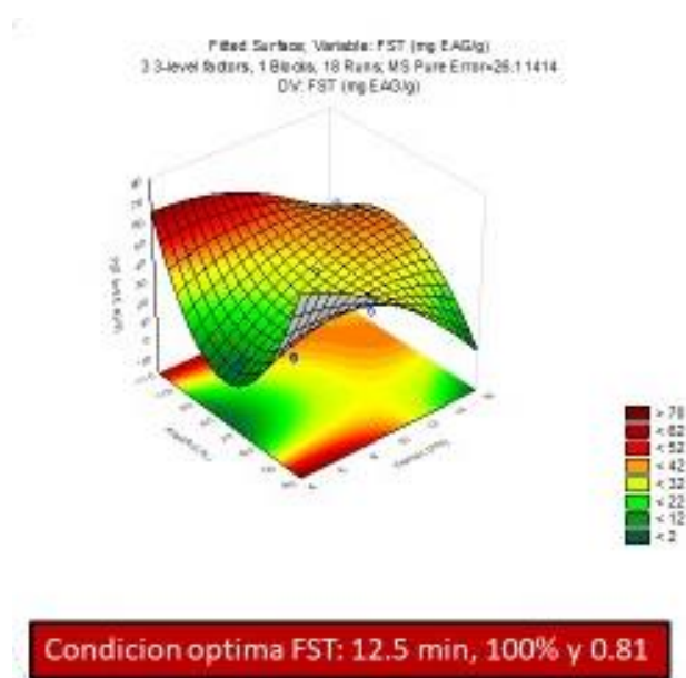
Figura 1.- Superficie de respuesta de capacidad antioxidante para DPPH en cascara de guamuchil.
