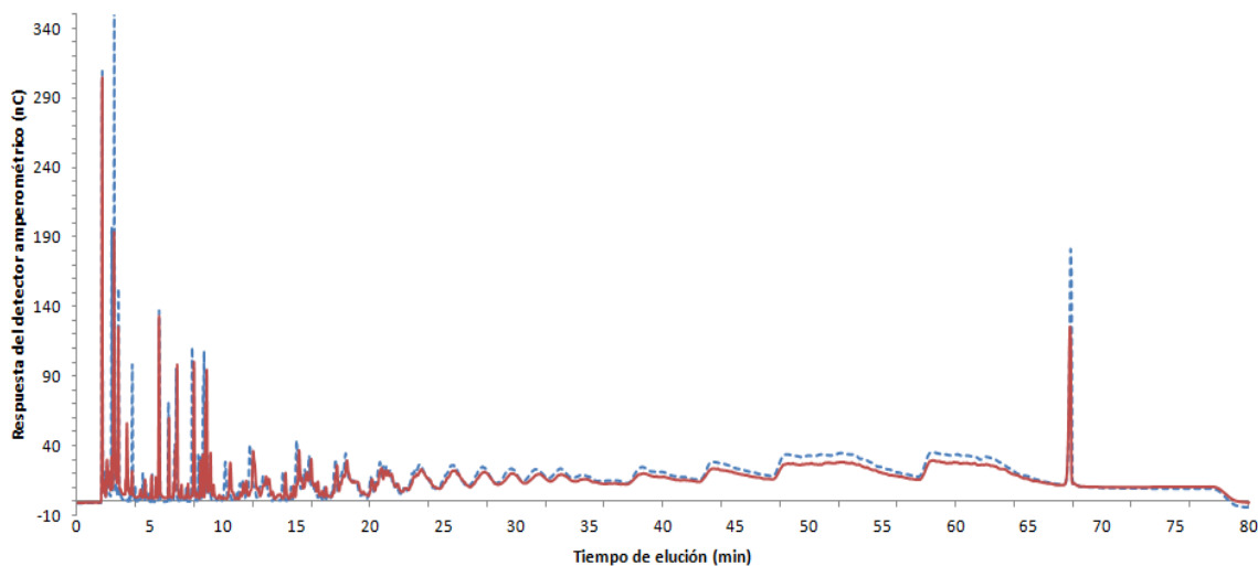
Figura 2. Perfil cromatográfico de alimentación (---) y retenido (—) obtenido en proceso de filtración empleando una membrana de 1000 Da.
