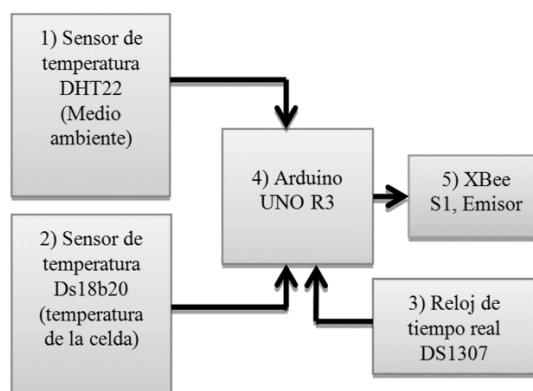
Figura 1. Esquema de la tarjeta de adquisición de datos con la que se trabajó
