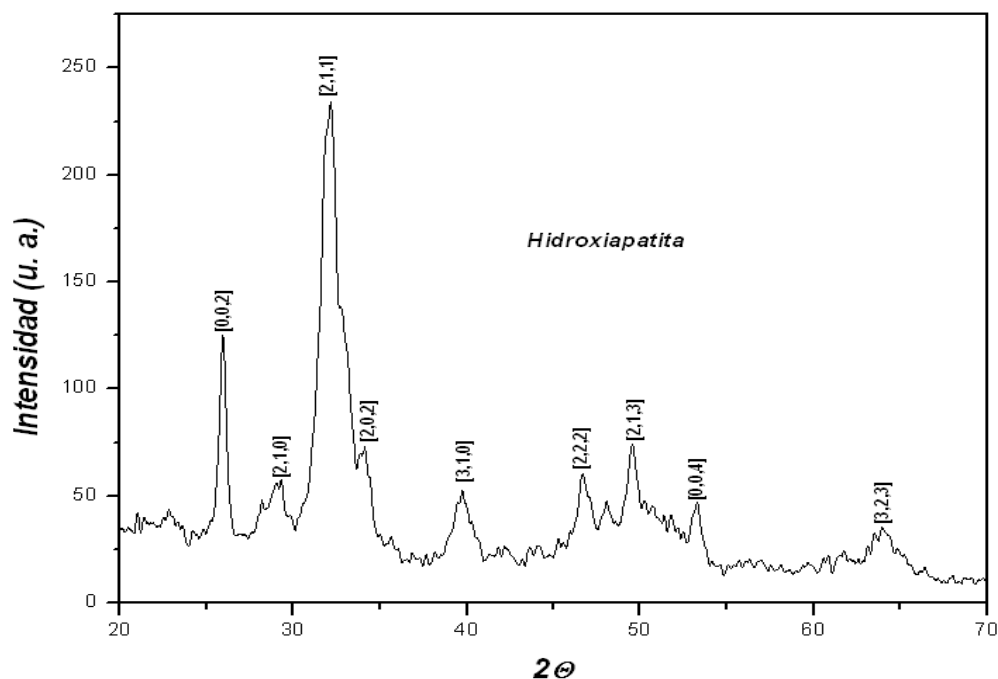
Figura 4. Difractograma de Hidroxiapatita (HA)
