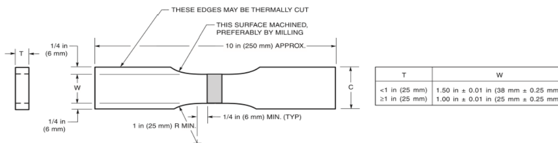
Figura 4: Especificaciones de las dimensiones de la probeta sometida a prueba de tensión por la American Welding Society (AWS), (Society, 2000).
