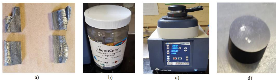
Figura 9: Realización de portamuestras: a) Corte en extremo periféricos del área soldada, b) Baquelita utilizada para portamuestra, c) Máquina de portamuestra BUEHLER en proceso y d) Proceso de portamuestra terminado
