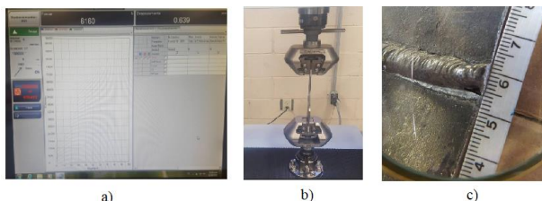
Figura 8: Prueba de tensión: a) Software Trapezium X, b) Máquina de ensayos universal SHIMADZU aplicando una carga de tracción y c) Fractura en probeta biselada con ángulos de 45°
