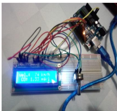
Figura No. 1 Arduino con display
