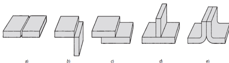
Figura 1: Cinco tipos de uniones soldadas: a) empalmada, b) de esquina, c) superpuesta, d) en te y e) de bordes.
