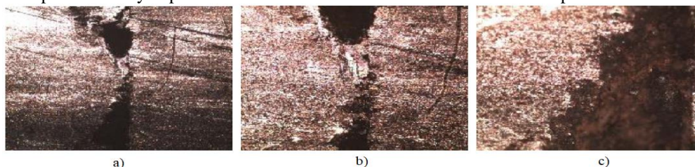
Figura 3: Falta de fusión entre el material base y el metal depositado, observada en el microscopio: a) lente 20X, b) lente 50X y c) lente 100X.
