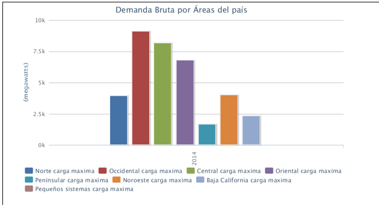
Fig. 1. Demanda de energía en Mega-watts por regiones en México
