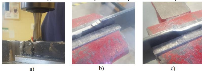
Figura 7: Procesos de Maquinado: a) Fresado de Probetas, b) Desbaste en área del Fillet y c) Limado del fillet
