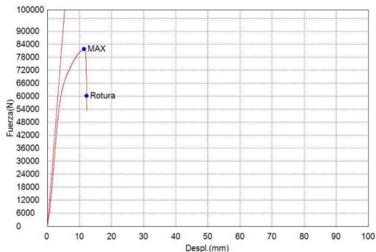
Gráfica 1: Diagrama esfuerzo-deformación elaborado por el software Trapezium X, mediante la realización del ensayo de tensión sobre la probeta con biseladas de 45° en ambas vistas de los extremos interiores.
