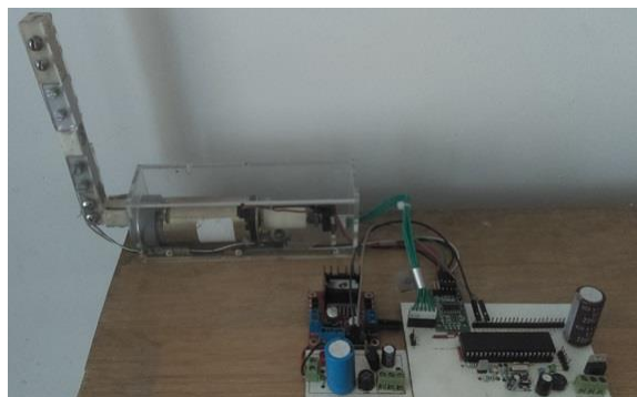
Figura 6. Sistema háptico de 1DOF.
