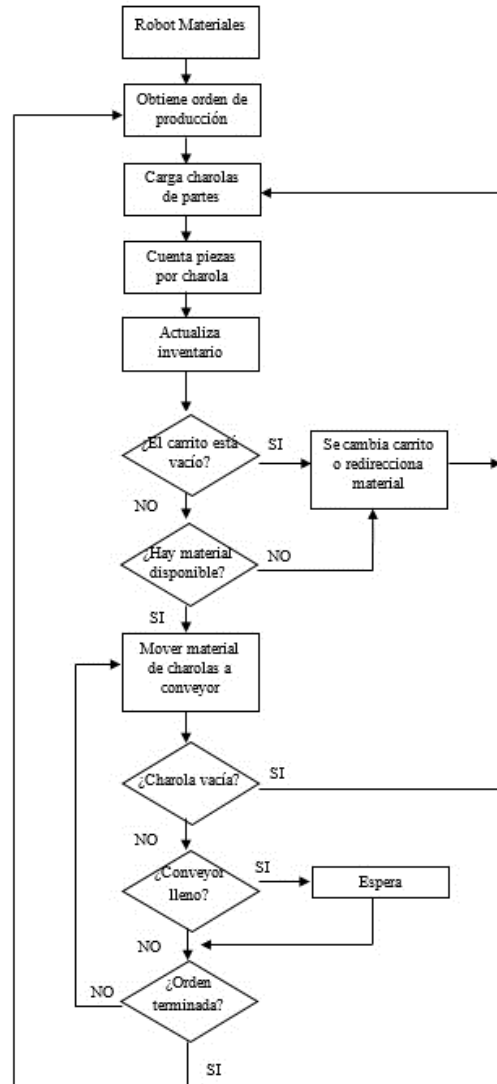
Figura 4. Diagrama de flujo de robot de materiales
