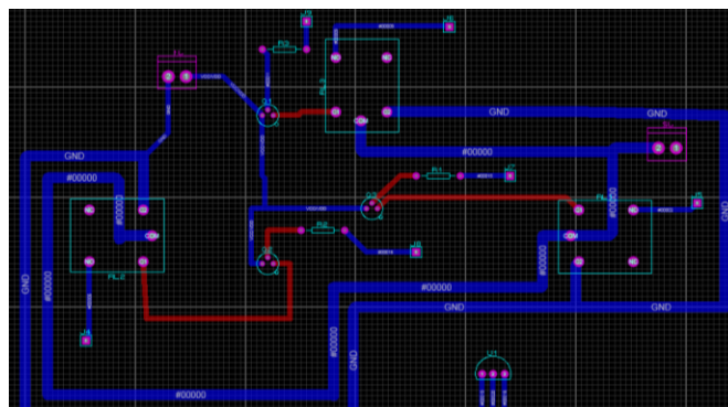
Figura 5. Diseño del circuito en PCB.
