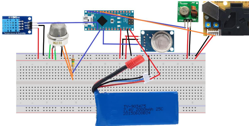
Figura 1. Implementación de los sensores y el transmisor con el Arduino nano
