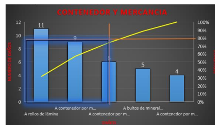
Gráfica 4. Pareto, Daños a Contenedores y mercancías
