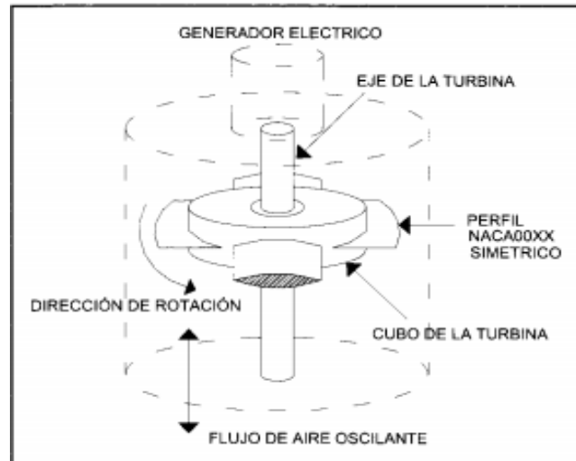
Fig. 02 Álabes
