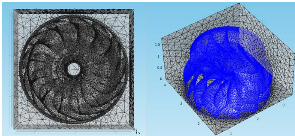
Figura 1. Malla en tres dimensiones de turbina y condiciones de frontera
