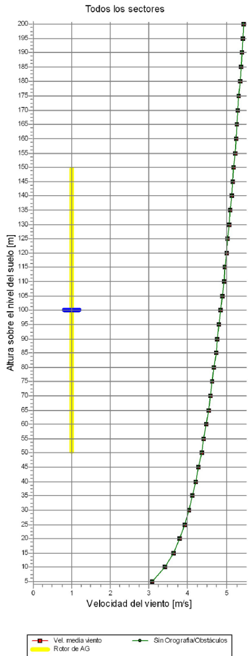
Figura 2. Perfil de velocidad del viento para Tepuxtepec, Michoacán.
