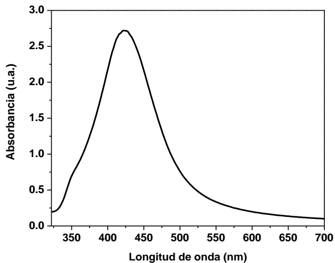
Figura 2. Espectro de absorción de la solución coloidal de partículas de Ag.
