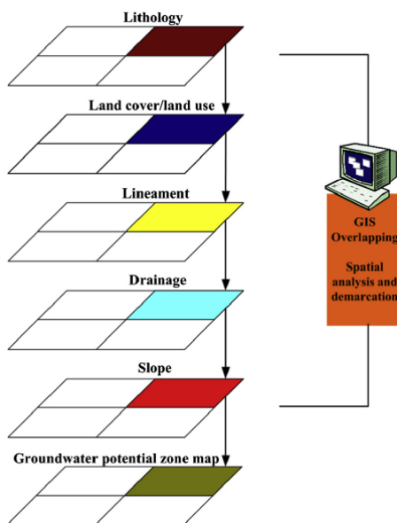
Figura 4. Tecnología SIG utilizada en integración espacial y análisis para delimitar zonas potenciales de recarga de aguas subterráneas (Yeh et al., 2015).
