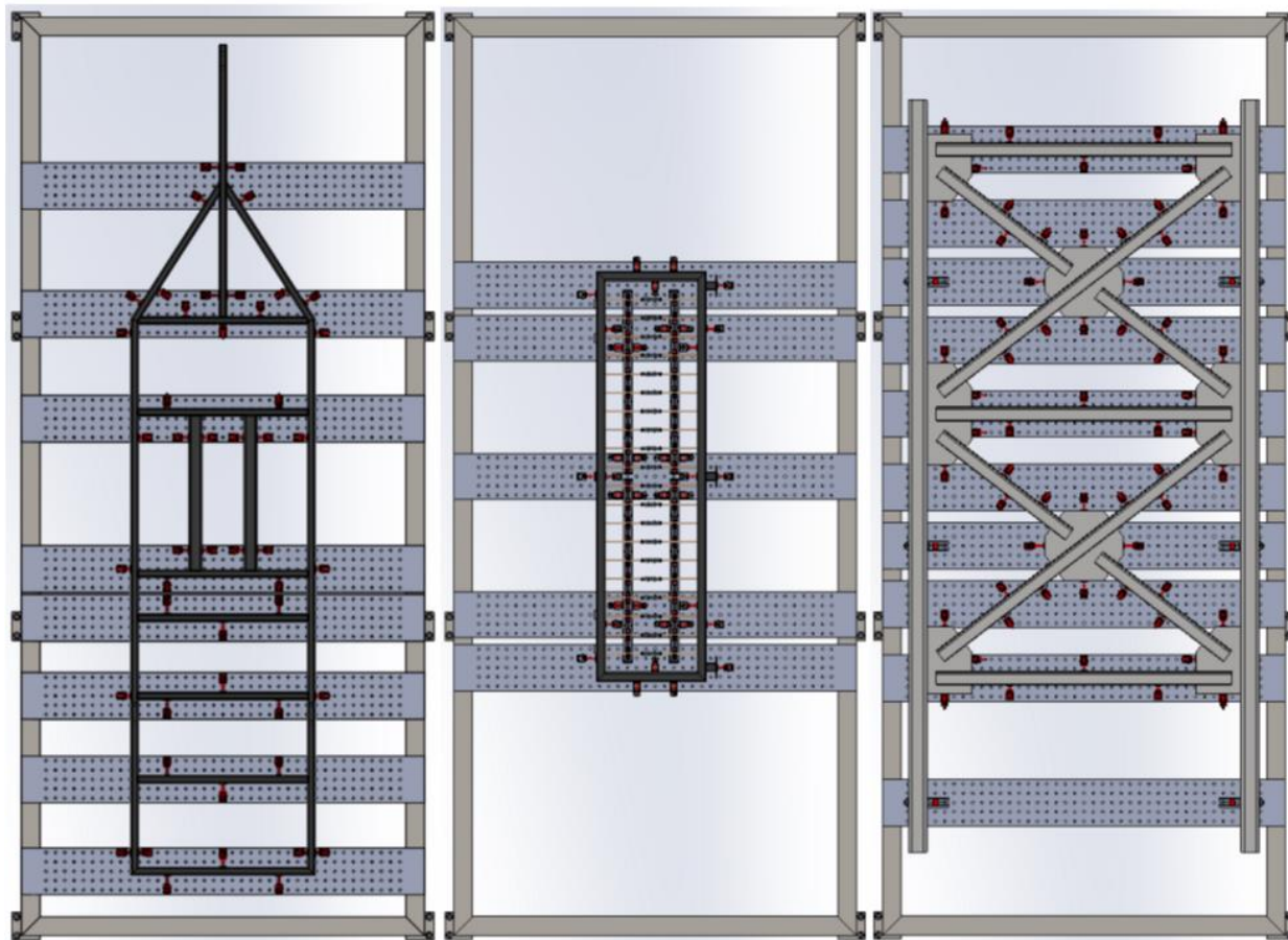
Figura 3 de izquierda a derecha, chasis de remolque, barandal, soporte estructural
