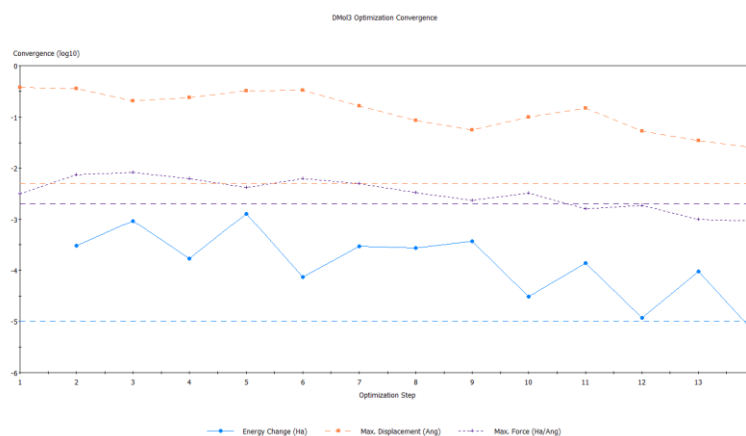
Figura 2. Optimización de la geometría de la lignina-Convergencia.
