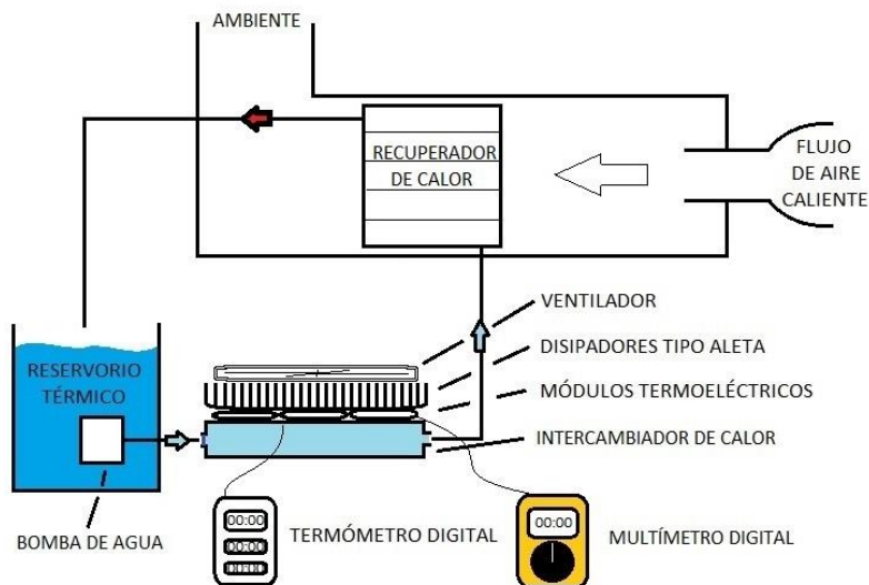
Figura 2. Esquema del Diseño del Sistema Experimental.
