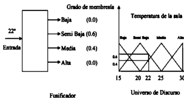
Figura 2. Entradas a un sistema difuso.
