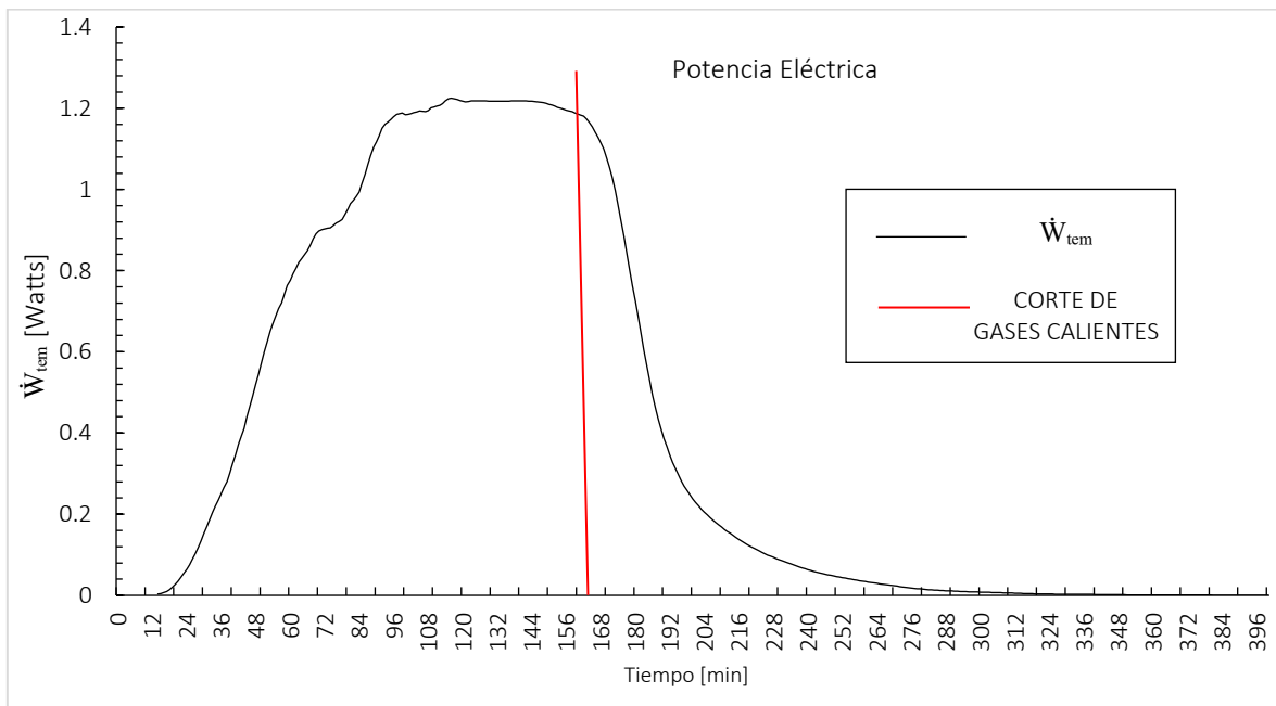
Figura 5. Potencia eléctrica ( \dot{W}_{te} ) generada a través del tiempo.
