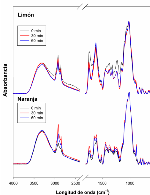
Figura 2. Análisis de Infrarrojo por transformada de Fourier de cáscaras de cítricos después de la extracción de polifenoles.
