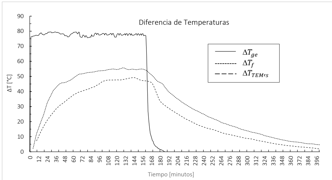
Figura 4. Diferencia de temperaturas ( \Delta T ) en el cosechador de energía.
