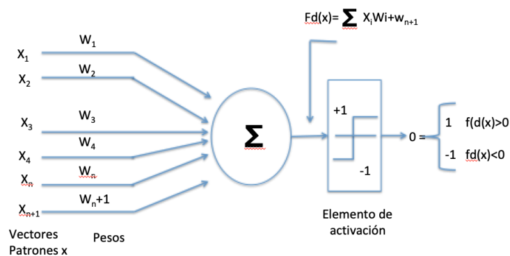
Figura 3. Modelo de perceptrón.
