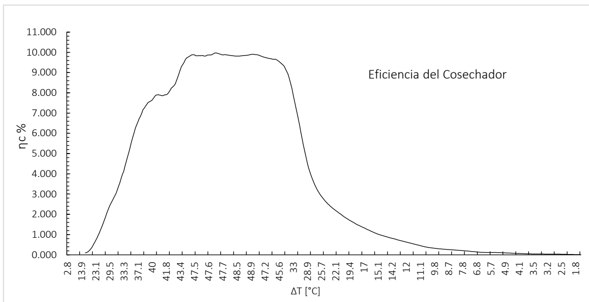
Figura 6. Eficiencia del Cosechador con respecto al diferencial de temperatura.
