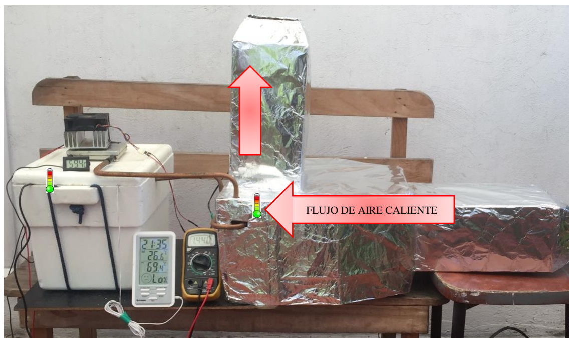
Figura 3. Imagen del arreglo experimental y el equipo de medición.
