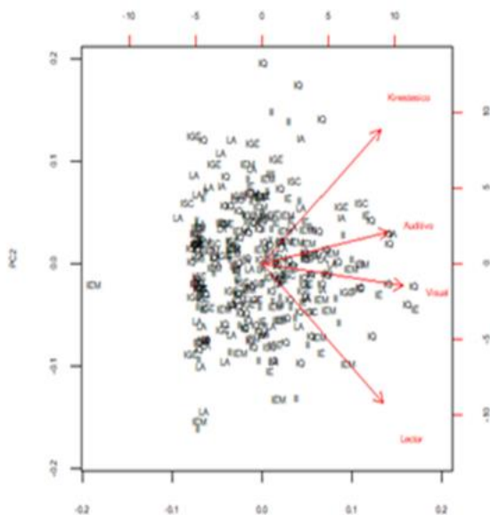
Gráfica 3. Biplot para los ejes 1-2. Instituto Tecnológico de Minatitlán 2018
