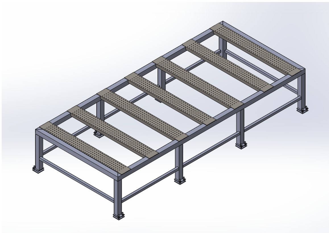
Figura 2 mesa de fijación
