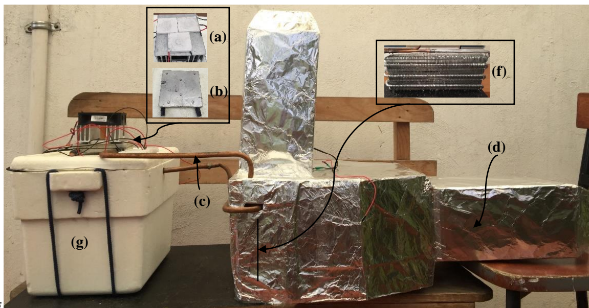
Figura 1. Configuración del Sistema: Cosechador de Energía.
