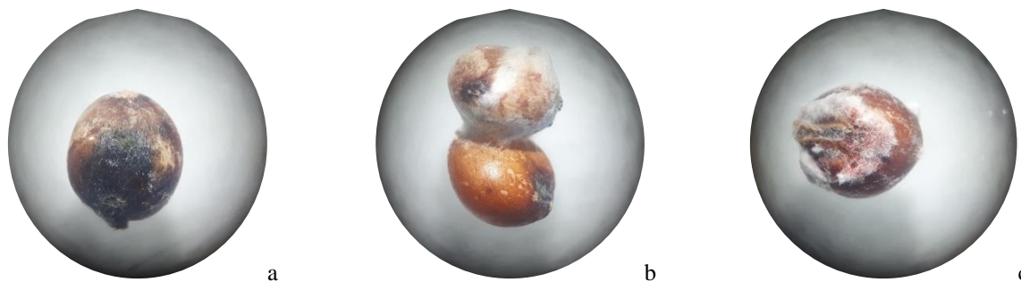
Figura 4. Granos de sorgo de la Granja "Marijo" vistos en estereoscopio. A simple vista es notable el desarrollo fúngico; a), b) y c) presentan infección aparentemente por diferentes cepas.
