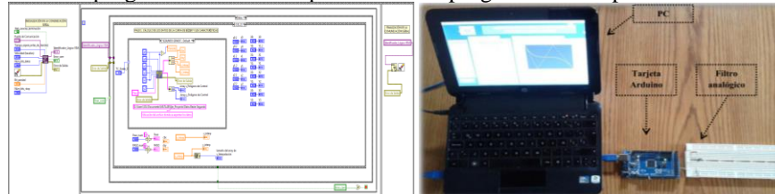
Figura 5. Diagrama de bloques en Labview de la interfaz de usuario y sistema final.
