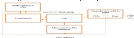
Figura 1. Diagrama de flujo del sistema.
