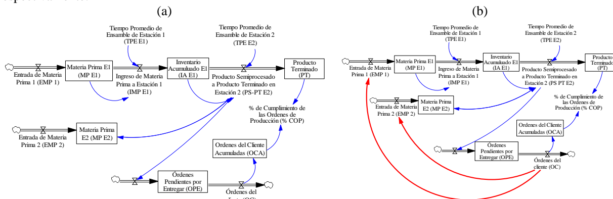
Figura 3: Modelo dinámico del proceso productivo (a) sistema Push y (b) sistema Pull
