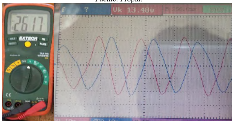
Figura 8. Medición de voltaje y forma de onda a la salida del estator.
