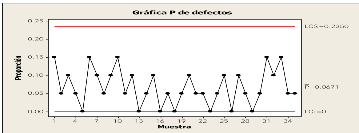
Gráfica 1: Gráfica de defectos
