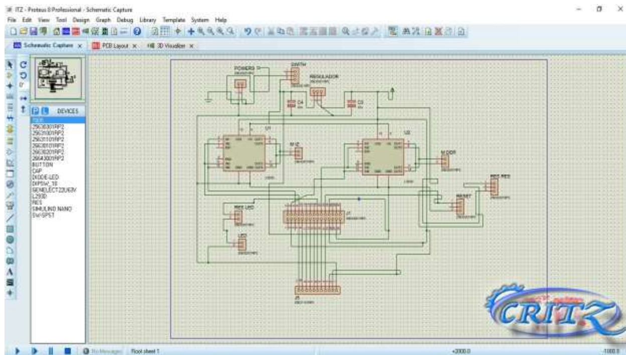
Figura 3. Diagrama de conexión del circuito y de sus componentes.
