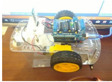
Figura 5 Prototipo Robot Móvil
