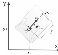
Figura 1 Representación del modelo cinemático
