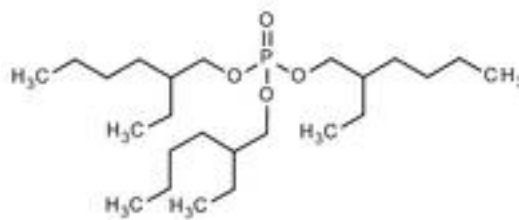
Figura 2. Estructura química del acarreador y plastificante tris(2-etil-hexil)fosfato.
