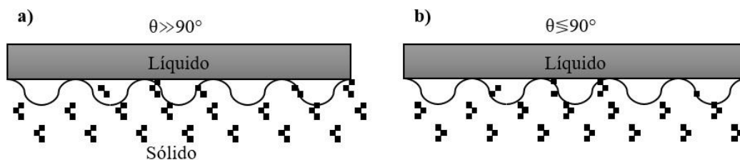
Figura 2. Configuración microscópica en interfaces sólido/líquido: a) Para \theta \gg 90^\circ , el líquido entra en contacto con la superficie rugosa del sólido solo en algunos puntos. b) Para valores de \theta inferiores a 90^\circ o superiores pero cercanos a este valor, existe un contacto íntimo en cualquier punto de la interfaz.
