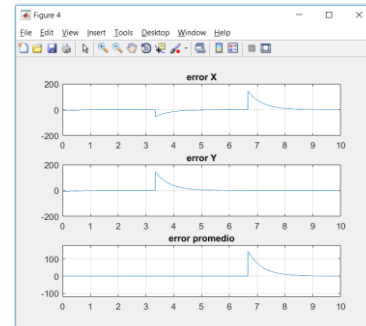
Figura 9 Errores de Posición
