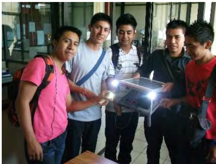
Figura 8. SSFV con panel de 10 W y lámparas de 1 W.
