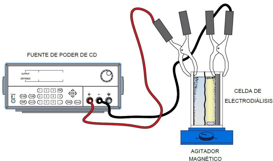
Figura 1. Esquema de la ejecución de las pruebas de electrodiálisis.
