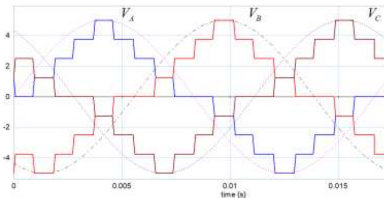
Figura 6. Dinámica de los voltajes trifásicos.
