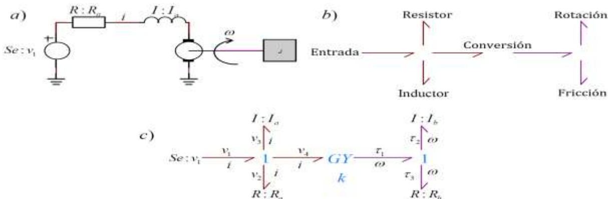
Figura 2. A) Modelo de un Motor de CC, b) Bond de intercambio de energía, c) Modelo en Bond Graph.
