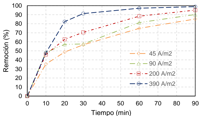
Figura 3. Porcentaje de remoción del hierro con una concentración inicial de 40 mg/L y un pH de 4 a diferentes densidades de corriente mediante el proceso de electrodiálisis.
