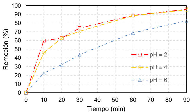
Figura 4. Porcentaje de remoción del hierro con una concentración inicial de 40 mg/L, una densidad de corriente de 200 A/m 2 y diferentes valores de pH.
