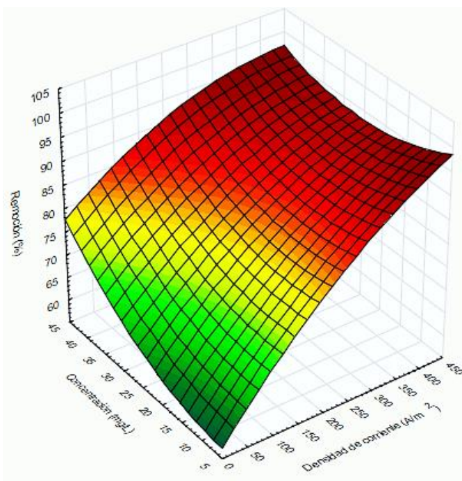
Figura 2. Gráfico tridimensional de remoción en función de la densidad de corriente y la concentración inicial de hierro con un pH de 4.
