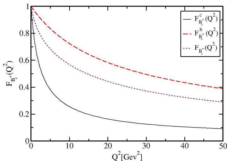
Figura 3. Factor de forma del mesón B_c^+ , compuesto por un quark pesado bottom ( b ) y un quark pesado charm ( c ). Se muestran también los valores individuales para cada quark.
