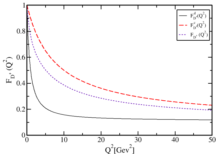
Figura 1. Factor de forma del mesón D^+ , compuesto por un quark pesado charm ( c ) y un quark ligero down ( d ). Se muestran también los valores individuales para cada quark.
