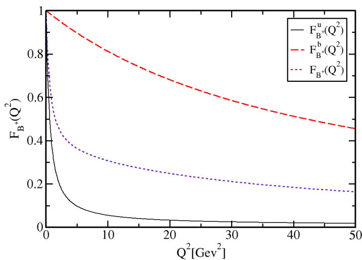
Figura 1. Factor de forma del mesón B^+ , compuesto por un quark pesado bottom ( b ) y un quark ligero up ( u ). Se muestran también los valores individuales para cada quark.
