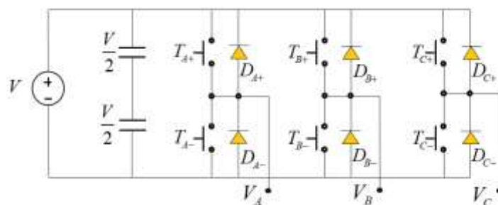
Figura 3. Inversor Trifásico.
