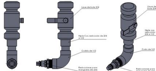
Figura 8. Conexión rápida de aire a presión a sistema.
