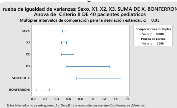
Gráfica 4: Prueba de igualdad de varianza
