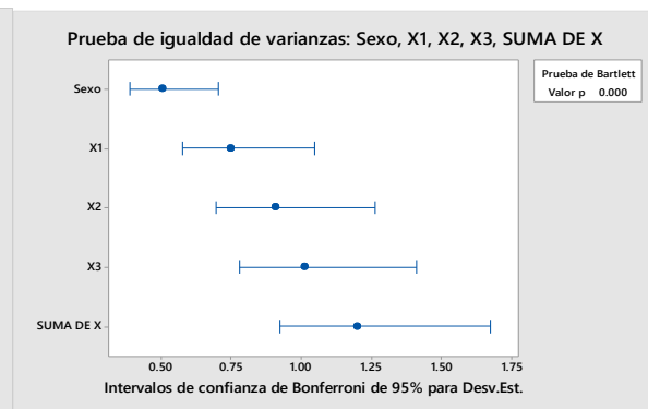
Gráfica 6: Prueba de varianza normal
