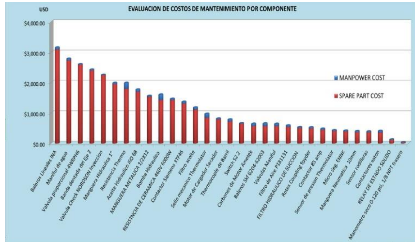
Figura 7 Análisis de costos de mantenimiento por parte.
