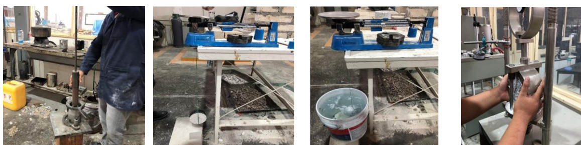
a) Elaboración de probetas b) Peso en el aire c) Peso en el agua d) Estabilidad Figura 4.- Procedimiento, estabilidad Marshall.
