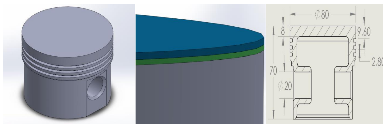
Figura 1. a) Geometría Pistón b) material cerámico y capa de enlace c) Vista sección de Pistón
