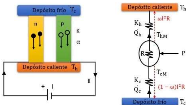
Figura 1. Esquema de un enfriador termoeléctrico (TEC)
