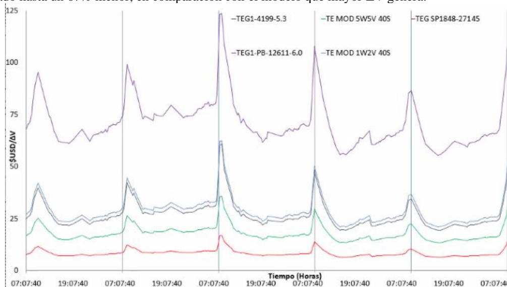
Figura 6. Relación costo & generación de diferencia de potencial de módulos termoeléctricos comerciales con respecto al tiempo.
