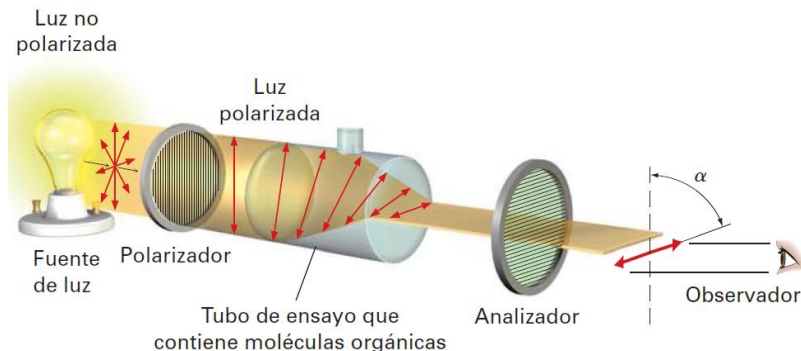
Figura 3. Funcionamiento básico de la polarimetría.
