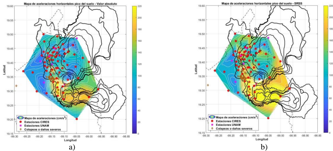
Figura 2. Mapa de aceleraciones horizontales pico en la zona instrumentada. a) PGA Absoluto, b) PGA SRSS
