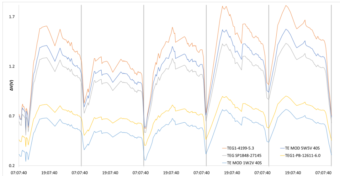
Figura 5. Generación de diferencia de potencial de módulos termoeléctricos comerciales con respecto al tiempo; evaluados con la diferencia de temperaturas obtenidas de manera experimental en un termotanque con respecto al ambiente, en temporada de invierno.
