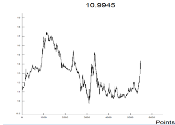
Gráfica 8 del variograma en BENOIT™ Elaboración propia
