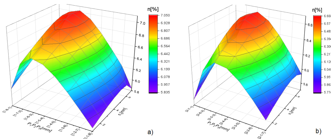
Figura 5. Eficiencia del STEG como función de la longitud de los termoelementos, para un modelo con 3 segmentos en el termoelemento tipo p con el modelo TDPM, a) L_{p1} = 1mm y b) L_{p1} = 2mm .
