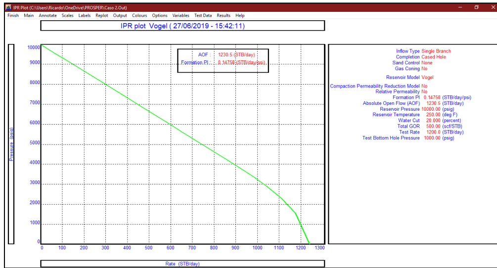
Figura 4. Curva IPR del caso de estudio.
