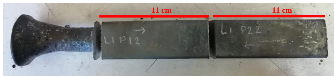
Fig. 3. Lingote seccionado.
