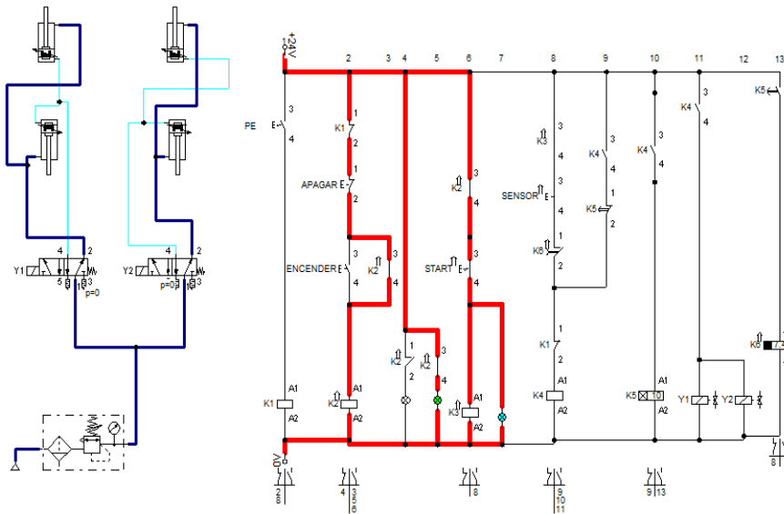
Figura 15 Activación de las electroválvulas
