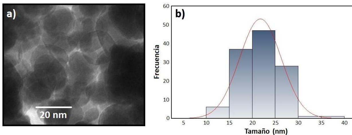
Figura 2. Resultados de TEM de las NPs de \text{Fe}_3\text{O}_4 -PVP, operado a 100 kV y 100,000. X a) Fotomicrografía; b) Histograma.
