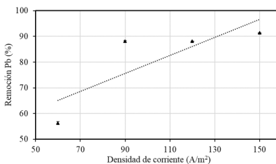
Figura 3. Porcentaje de Remoción Final de Plomo en función de la densidad de corriente. Velocidad de recirculación: 80 ml/min; Concentración de NaCl: 5 g/L
