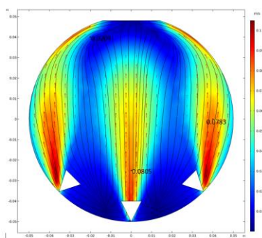
Figura 4 Distribución de velocidades con \alpha=0^\circ
