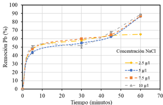
Figura 7. Cinética de Remoción de Plomo en función de la concentración de NaCl. Densidad de corriente: 120 A/m 2 ; Velocidad de recirculación: 80 ml/min
