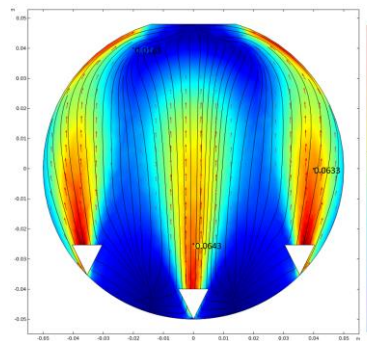
Figura 6 Distribución de velocidades con \alpha=45^\circ
