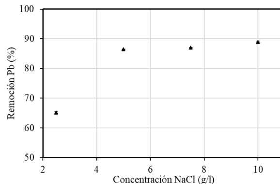
Figura 8. Porcentaje de Remoción Final de Plomo en función de la concentración de NaCl. Densidad de corriente: 120 A/m 2 ; Velocidad de recirculación: 80 ml/min
