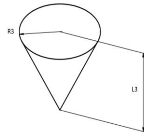
Figura 3 Dimensiones de los deflectores
