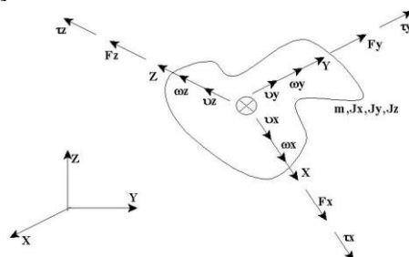
Figura 1. Cuerpo en multipuerto 3-D general.
