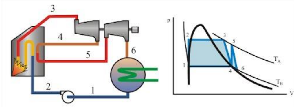
Figura 8. Ciclo Rankine
