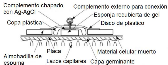
Figura 1. Representación gráfica del electrodo flotante.
