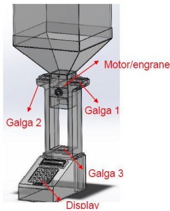
Figura 3. Diseño dispensador
