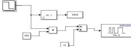
Figura 5 Lectura de la válvula de control
