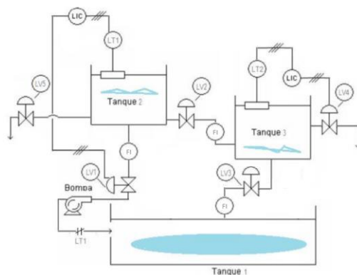
Figura 1. Sistema hidráulico propuesto.
