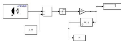
Figura 4 Lectura del sensor ultrasónico
