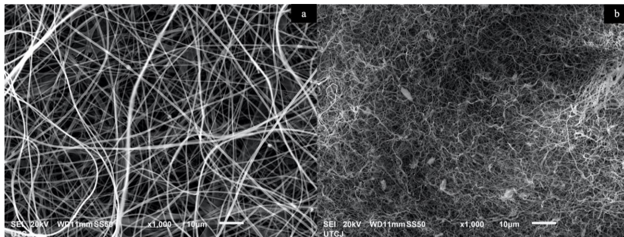
Figura 3. Micrografías SEM de las fibras de SiO 2 -HAp antes (a) y después (b) del tratamiento térmico.
