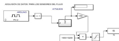
Figura 3 Lectura sensor de flujo efecto hall
