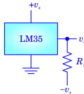
Figura 2. Configuración de conexión de escala completa de temperatura del sensor LM35.
