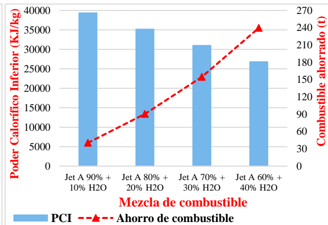
Figura 5. PCI vs Ahorro de combustible de 1918 motores V2500-A1 durante la fase de carreteo en la semana de control.
