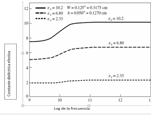
Figura 1. Comportamiento de la constante dieléctrica efectiva contra la frecuencia. Fuente [11].
