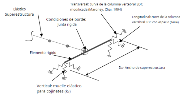
Figura 1-7 Modelo de estribo simplificado
