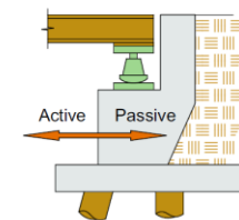
Figura 1- 5 Definición del relleno longitudinal del estribo.
