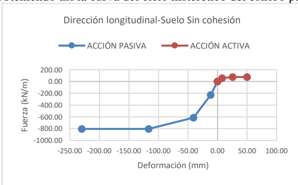
Figura 1- 10 Curva en dirección longitudinal de suelo sin cohesión
