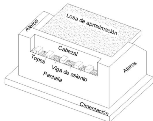
Figura 1- 1 Partes de un estribo
