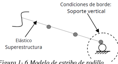
Figura 1-6 Modelo de estribo de rodillo
