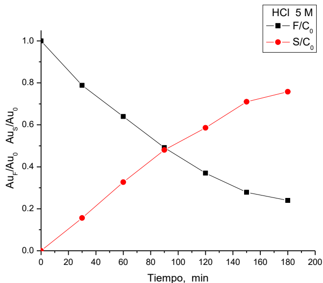
Figura 5. Transporte de Au(III) a través de la membrana. Alimentación: Au(III) en HCl 5 M. Recuperación: NaCl 0.1 M. Ciclo de operación: 180 min.
