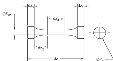
Figura 5. Geometría de la Probeta
