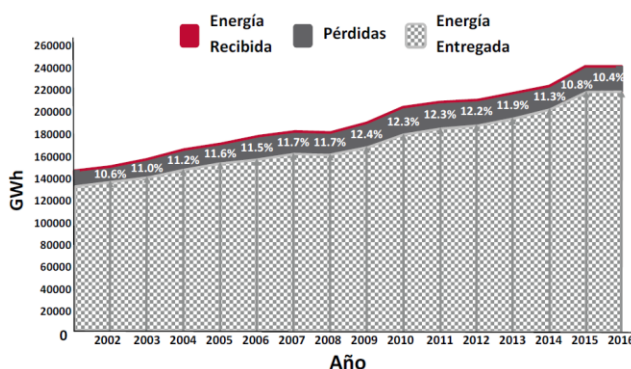
Figura 1. Pérdidas de energía (GWh) en Distribución 2002-2016 Interior de la República.
