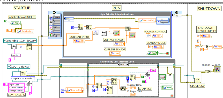
Figura 7. Diagrama de bloques con la implementación del módulo de Tiempo-Real
