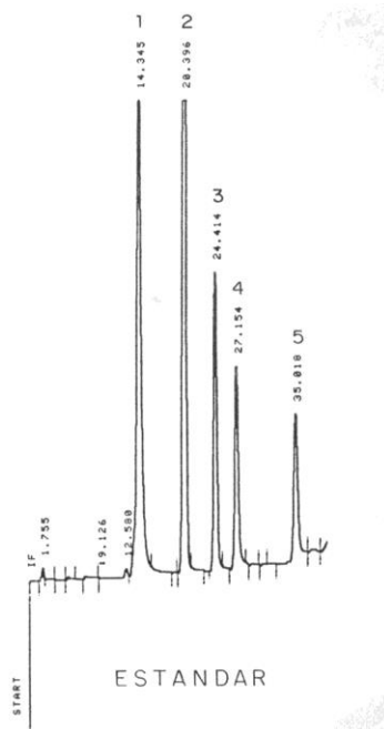
Figura 2. Separación de la mezcla de fenoles con gradiente de elución usando como fase móvil: Fase A: acetonitrilo-agua(pH 4.5) (15:85) v/v, y la fase B: acetonitrilo-agua(pH 4.5) (70:30). Buffer de ácido acético- acetato de sodio. El tiempo de separación es de aproximadamente 40 minutos. Flujo 1 mL/min, detector UV. Sensibilidad 0.05 AUFS. El orden de elución de los analitos es: 1) 4,6-dinitro-2-metilfenol, 2) 2,4-dimetilfenol, 3) 4-cloro-3-metilfenol, 4) 2,4-diclorofenol, 5) 2,4,6-triclorofenol y 6) pentaclorofenol. El gradiente usado es el siguiente:
