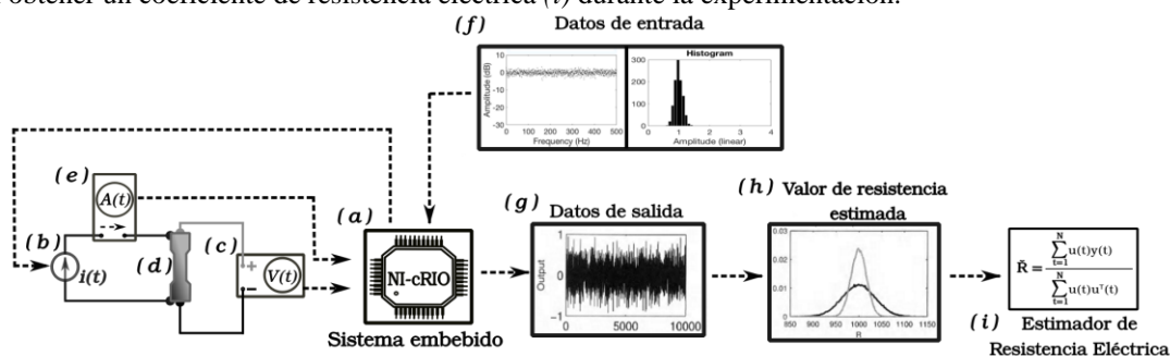
Figura 4. Metodología del estimador de propiedades eléctricas
