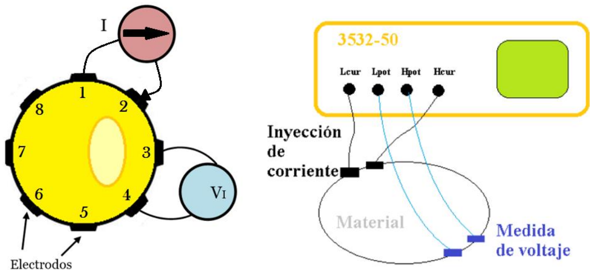
Figura 2. Inyección adyacente. Medición a 4 puntas con el medidor de impedancias.
