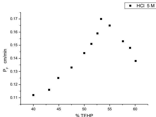
Figura 4. Variación de la permeabilidad ( P_F ) con respecto a la concentración de TEHP, tris(2-etil-hexil)fosfato, para la recuperación de oro a través de la membrana.
