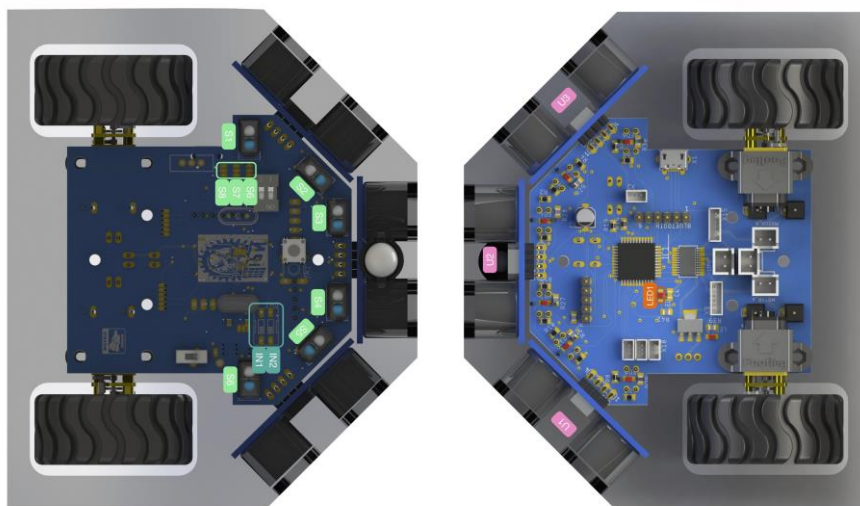
Figura 2. Vistas inferior, superior e isométrica del robot móvil en render 3D.
