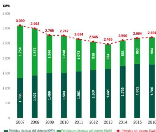
Figura 2. Pérdidas de energía eléctrica en los sistemas de distribución de Ecuador. Fuente (Duque & Romero, 2016)
