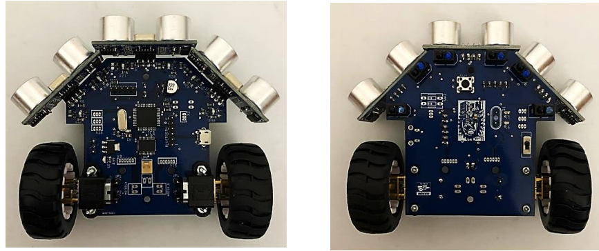
Figura 3. Vistas superior e inferior del robot móvil terminado.
