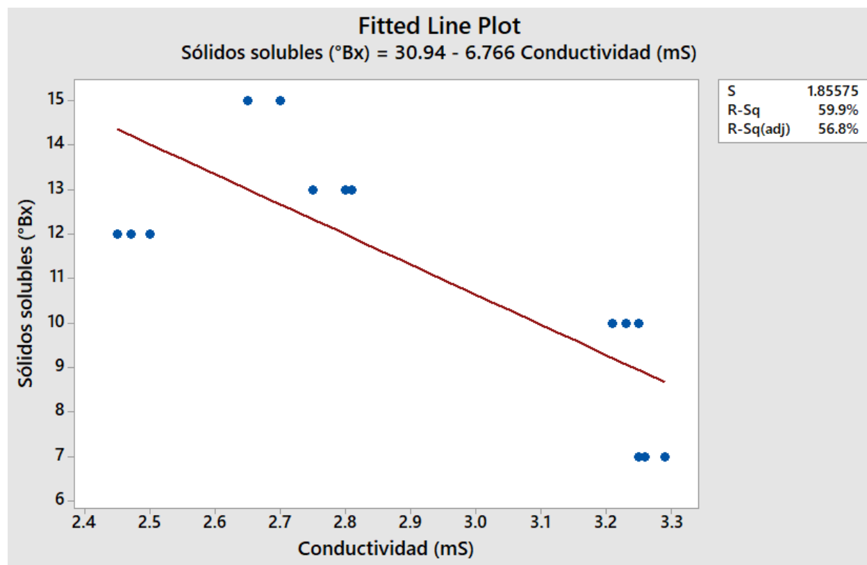
Figura 4. Regresión lineal de conductividad y sólidos solubles.
