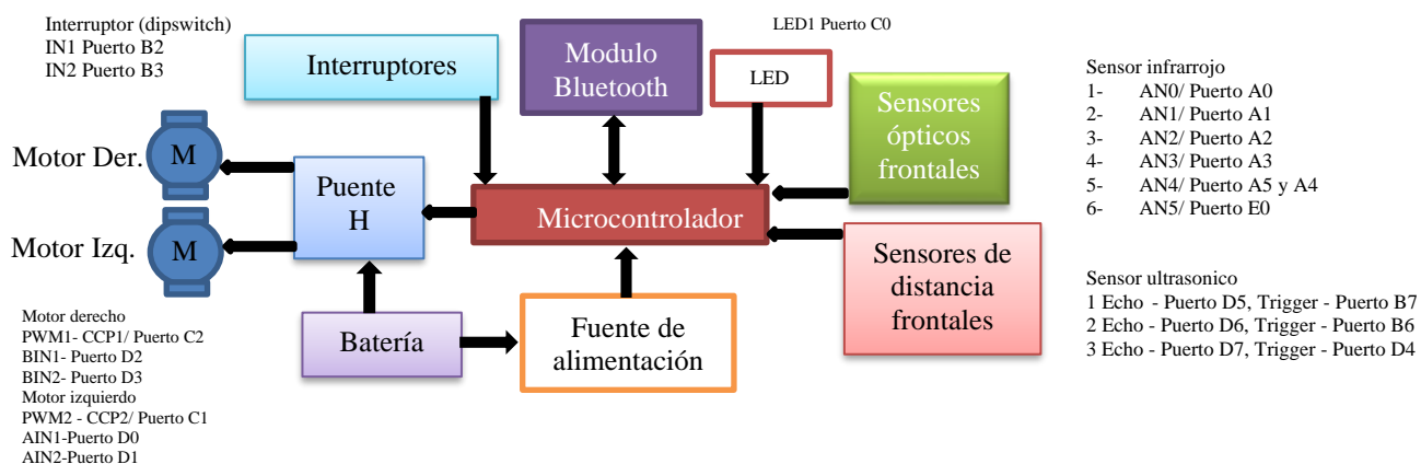
Figura 1. Diagrama a bloques del robot móvil y las terminales utilizadas.
