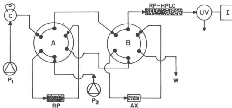
Figura 1. Sistema experimental en línea para efectuar la preconcentración, limpieza y análisis de fenoles. P 1 : sistema HPLC para gradiente binario, P 2 : bomba isocrática, A y B: válvulas de conmutación, C: inyector, W: deshechos, UV: detector ultravioleta , RP: precolumna polimérica de extracción, AX: precolumna aniónica de purificación, RP-HPLC: columna analítica C-18.
