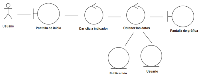
Figura 1. Caso de uso y diagrama de robustez CU01-Seleccionar indicador.
