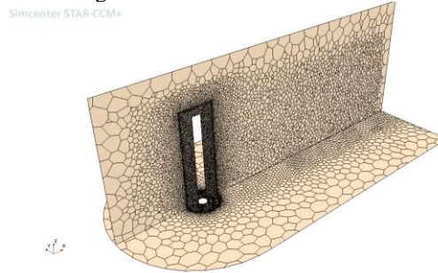
Figura 4 Malla del dominio tridimensional
